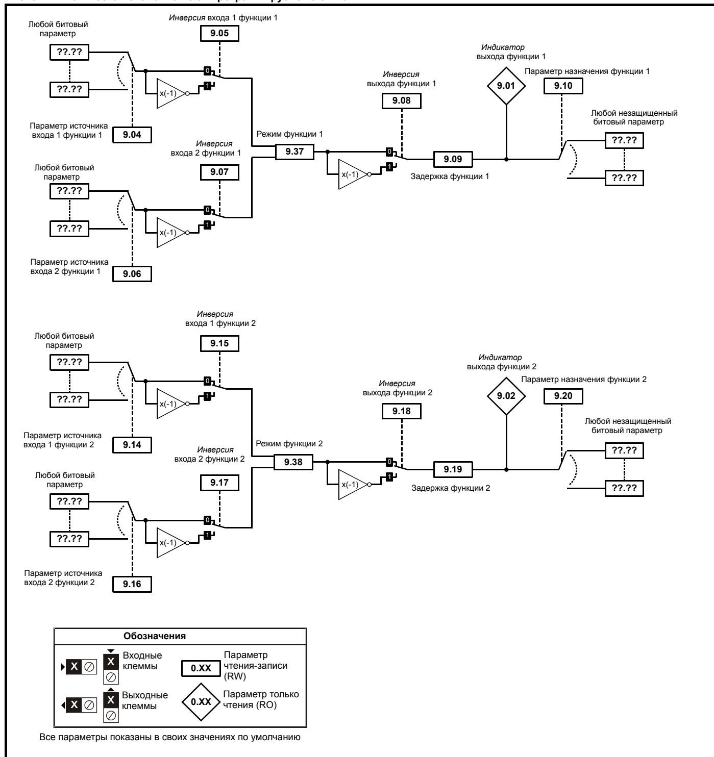
Рис. 8-12 Логическая схема Меню 9: Программируемая логика
