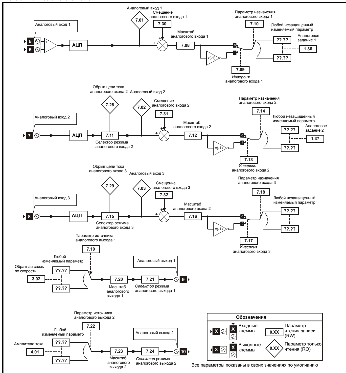
Рис. 8-8 Логическая схема Меню 7
