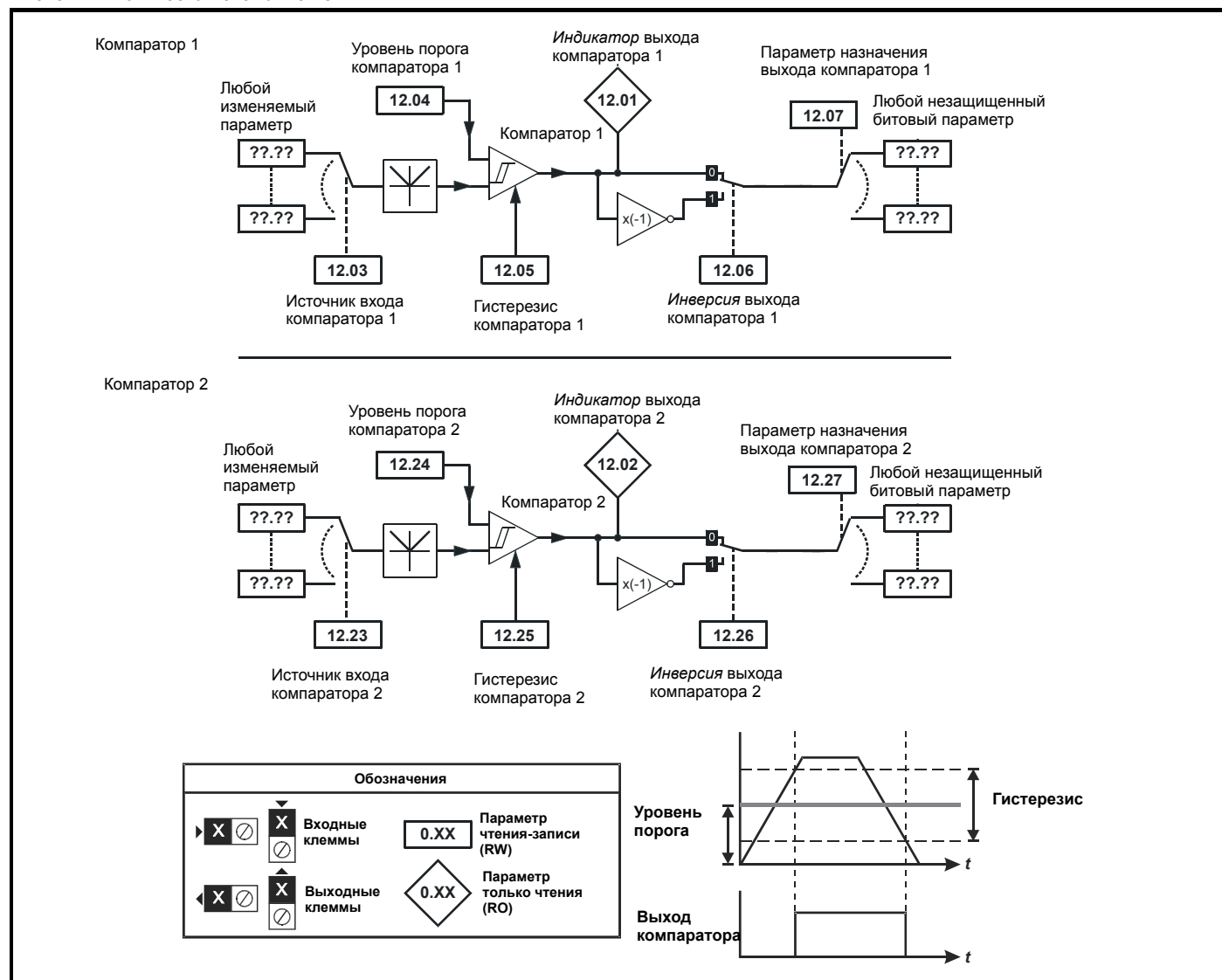
Рис. 8-14 Логическая схема Меню 12
