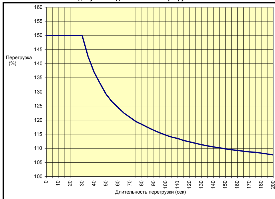
Рис. 2-1 Максимальная допустимая длительность перегрузки
