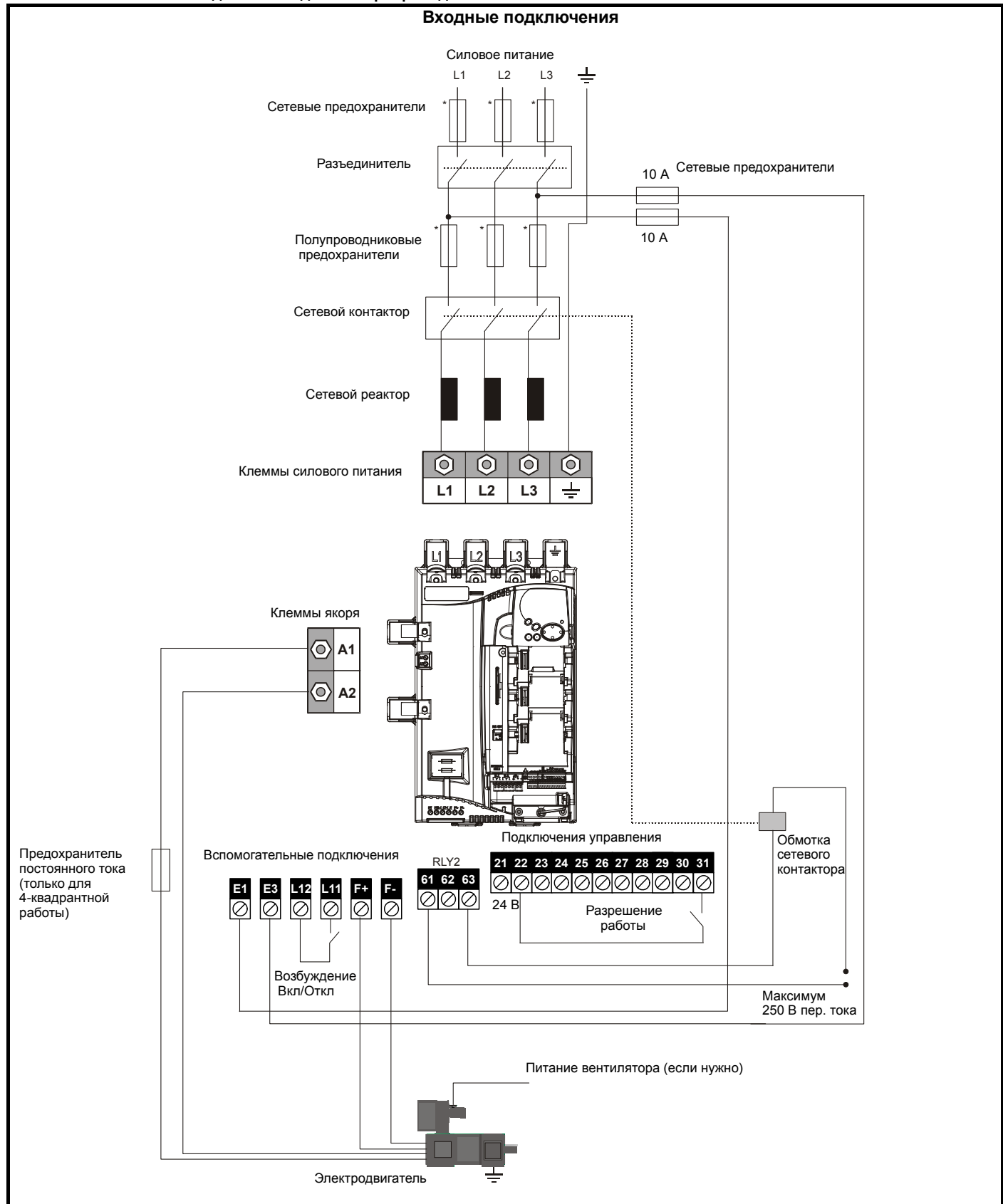
Рис. 4-1 Минимальные подключения для электропривода 480 В
