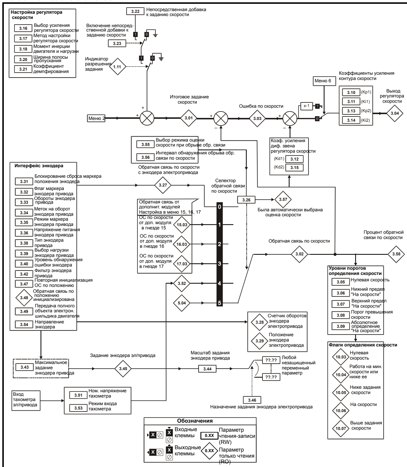
Рис. 8-3 Логическая схема Меню 3
