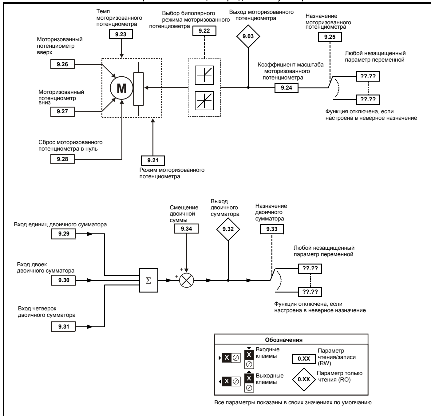
Рис. 8-13 Логическая схема Меню 9: Моторизованный потенциометр и двоичный сумматор
