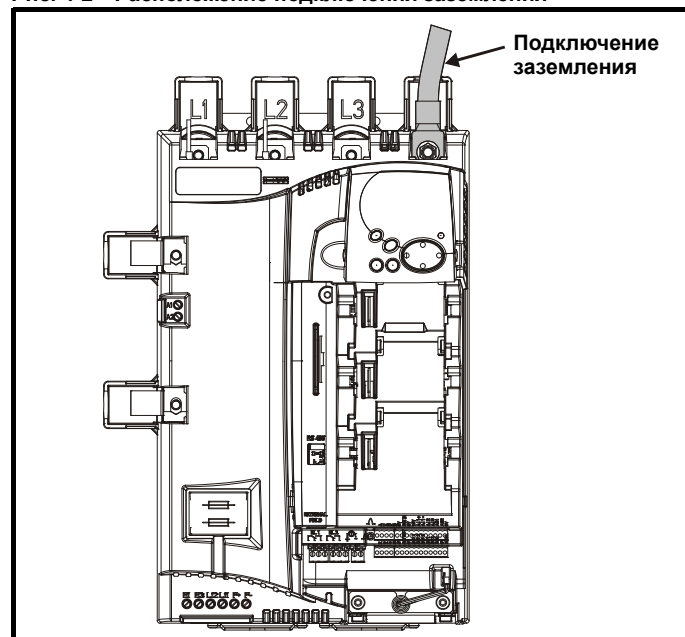
Рис. 4-2 Расположение подключения заземления
