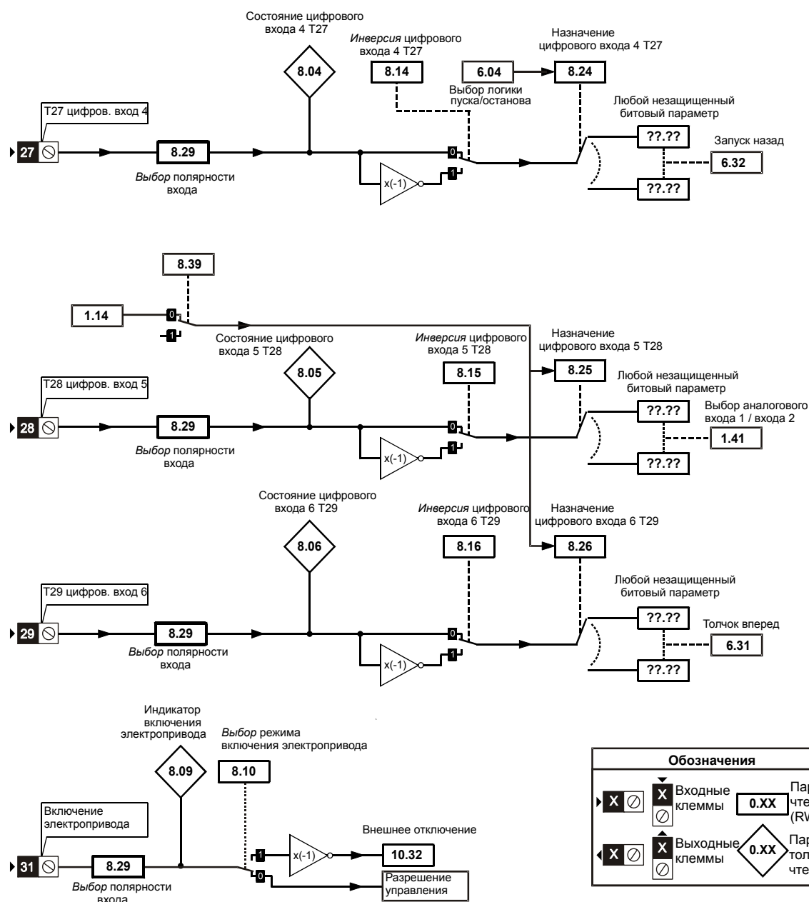
Рис. 8-10 Логическая схема Меню 8 (продолжение)
