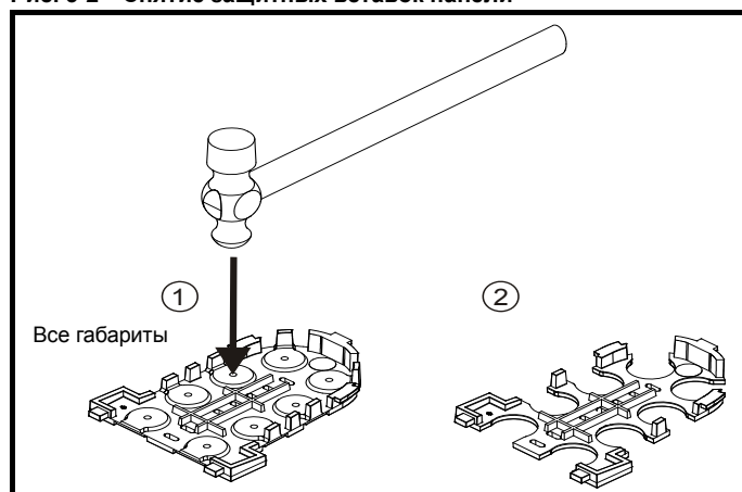
Рис. 3-2 Снятие защитных вставок панели
