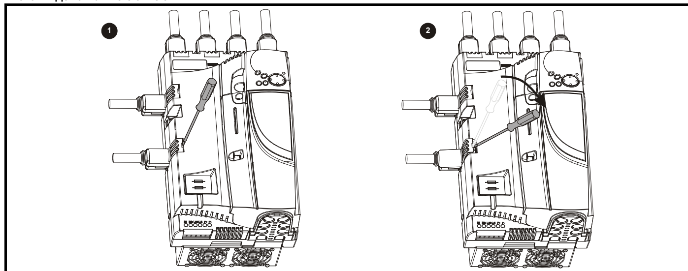
Рис. 3-7 Демонтаж чехлов клемм
