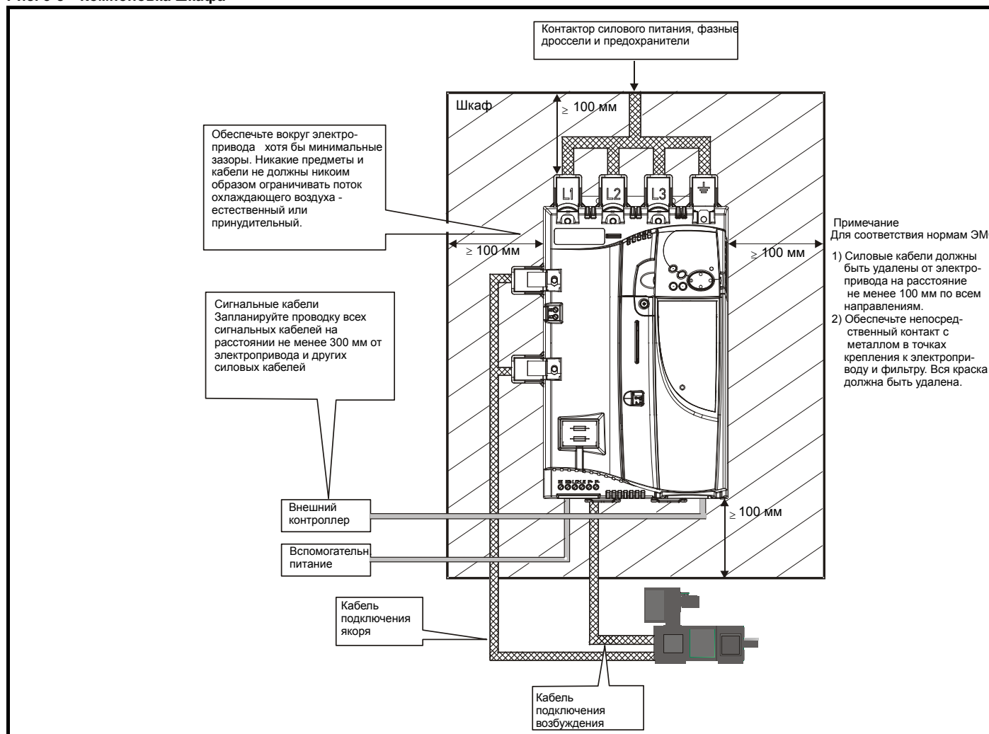
Рис. 3-8 Компоновка шкафа
