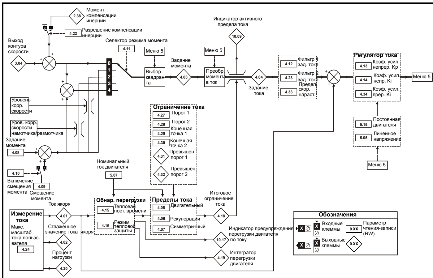
Рис. 8-4 Логическая схема Меню 4
