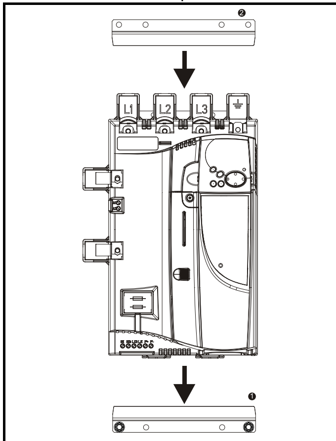
Рис. 3-5 Установка монтажного кронштейна
