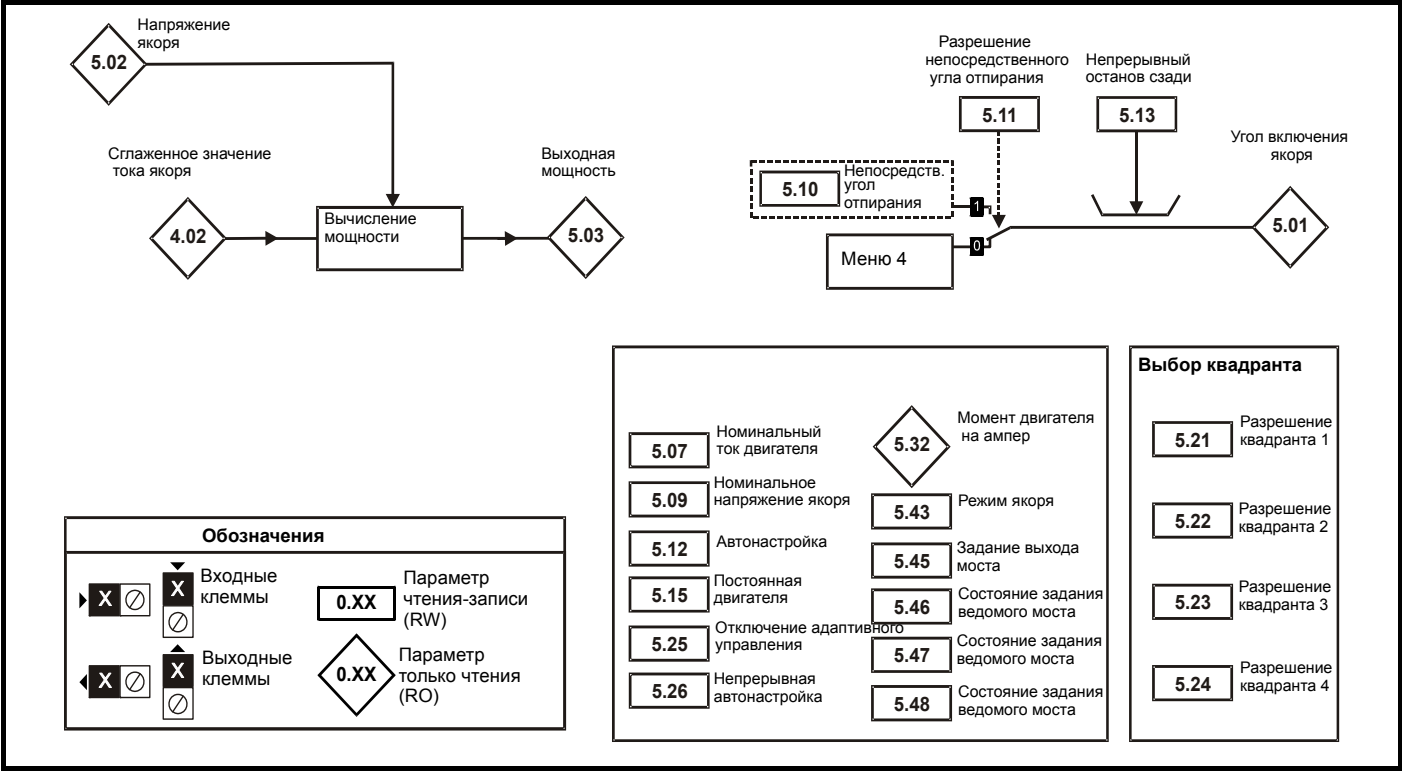
Рис. 8-5 Меню 5 - логическая схема управления якорем
