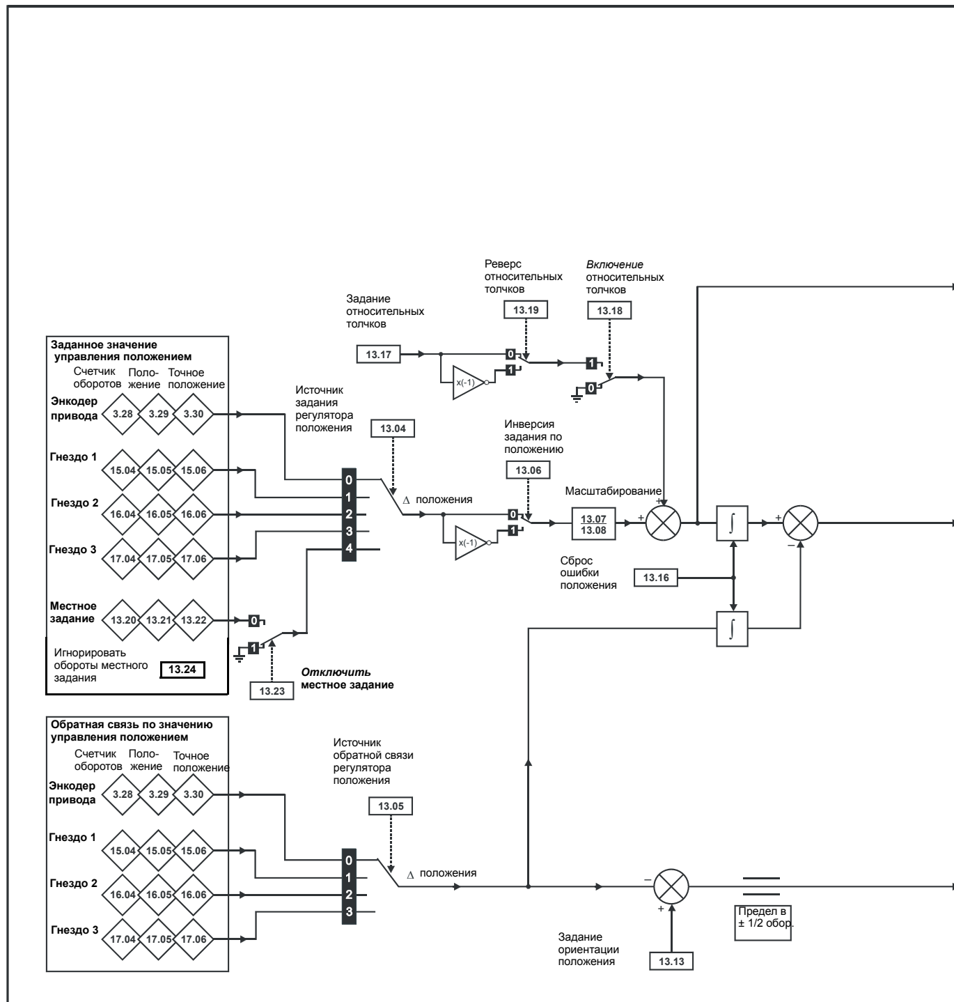
Рис. 8-17 Логическая схема Меню 13
