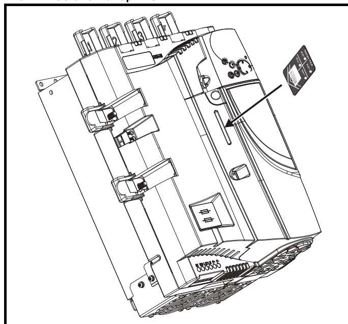
Рис. 7-1 Установка карты SMARTCARD
