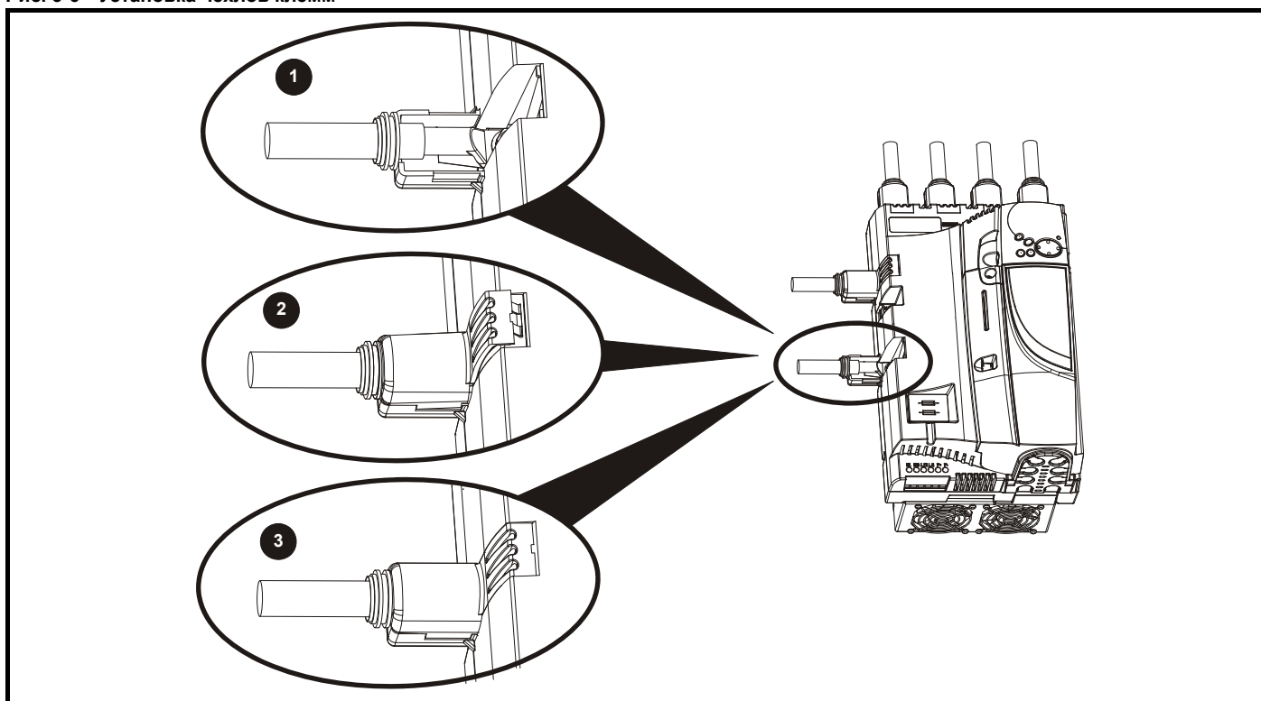
Рис. 3-6 Установка чехлов клемм
