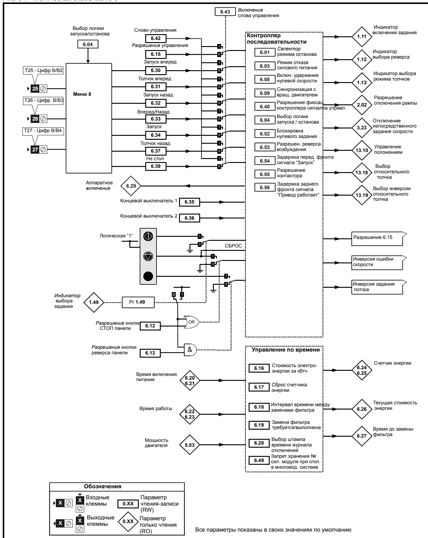
Рис. 8-7 Логическая схема Меню 6
