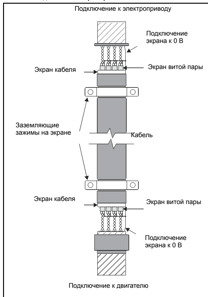
Рис. 4-4 Подключение экранированного кабеля
