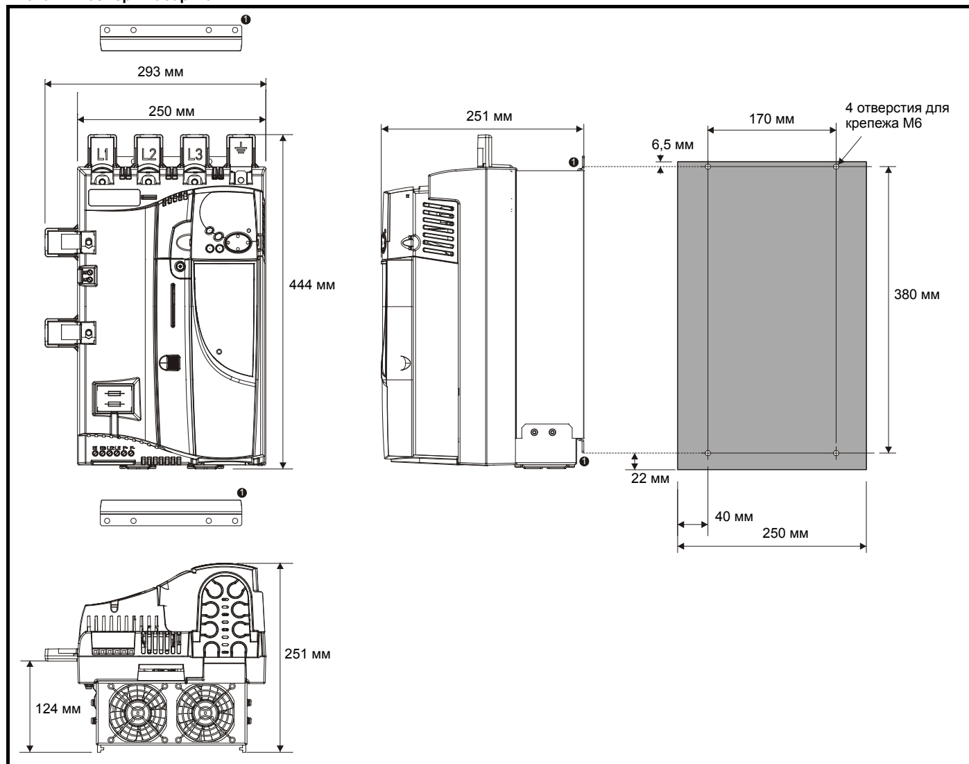
Рис. 3-4 Размеры габарита 1В
