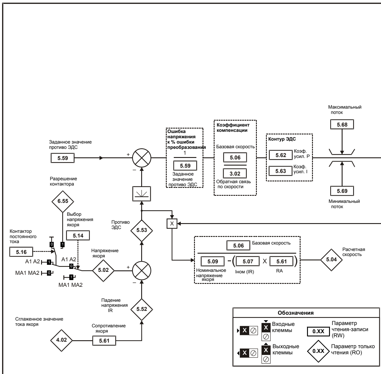
Рис. 8-6 Меню 5 - логическая схема управления якорем
