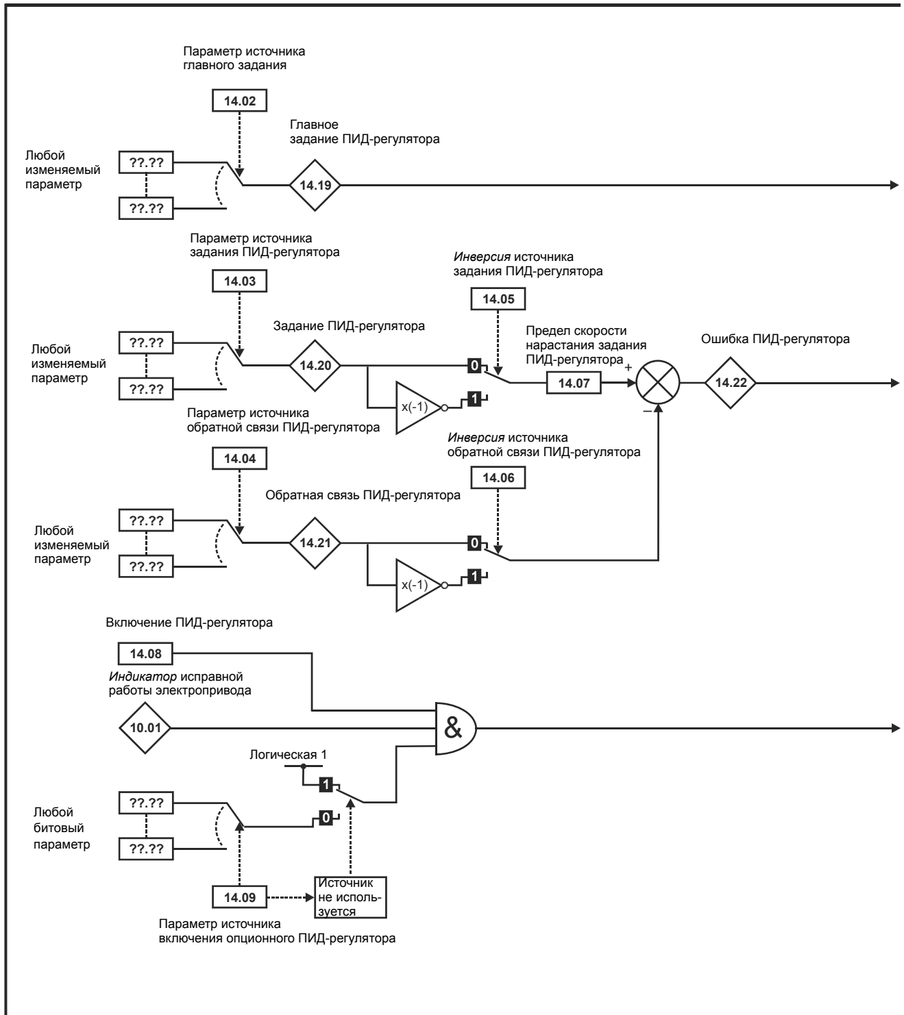
Рис. 8-18 Логическая схема Меню 14
