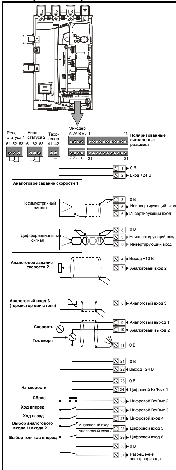
Рис. 4-5 Функции клемм по умолчанию
