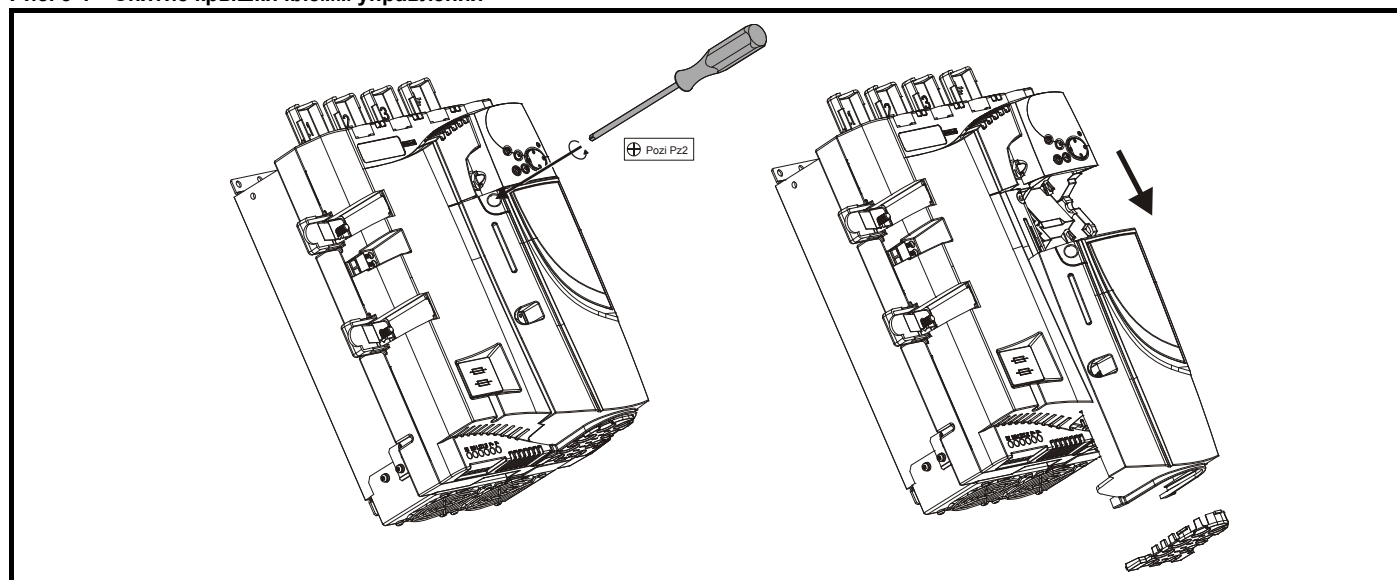
Рис. 3-1 Снятие крышки клемм управления
