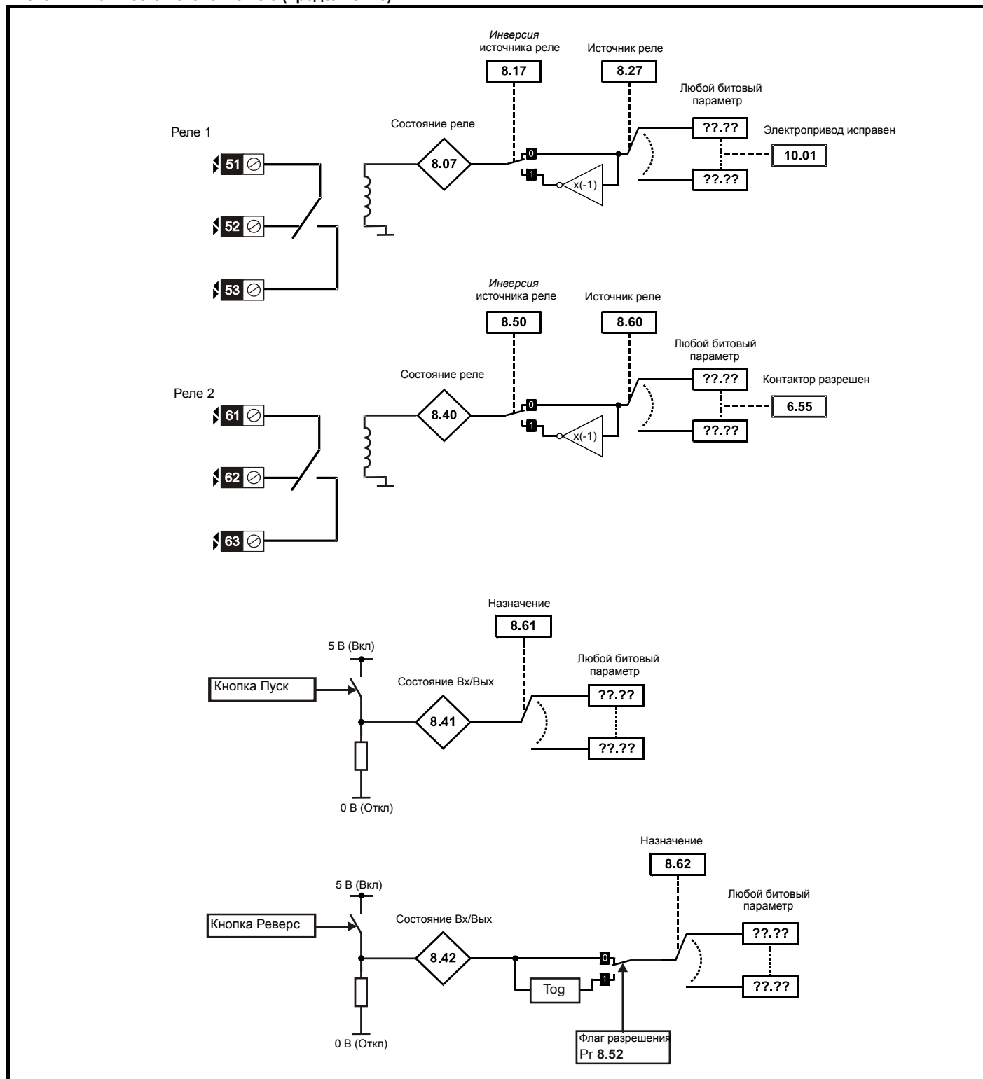
Рис. 8-11 Логическая схема Меню 8 (продолжение)
