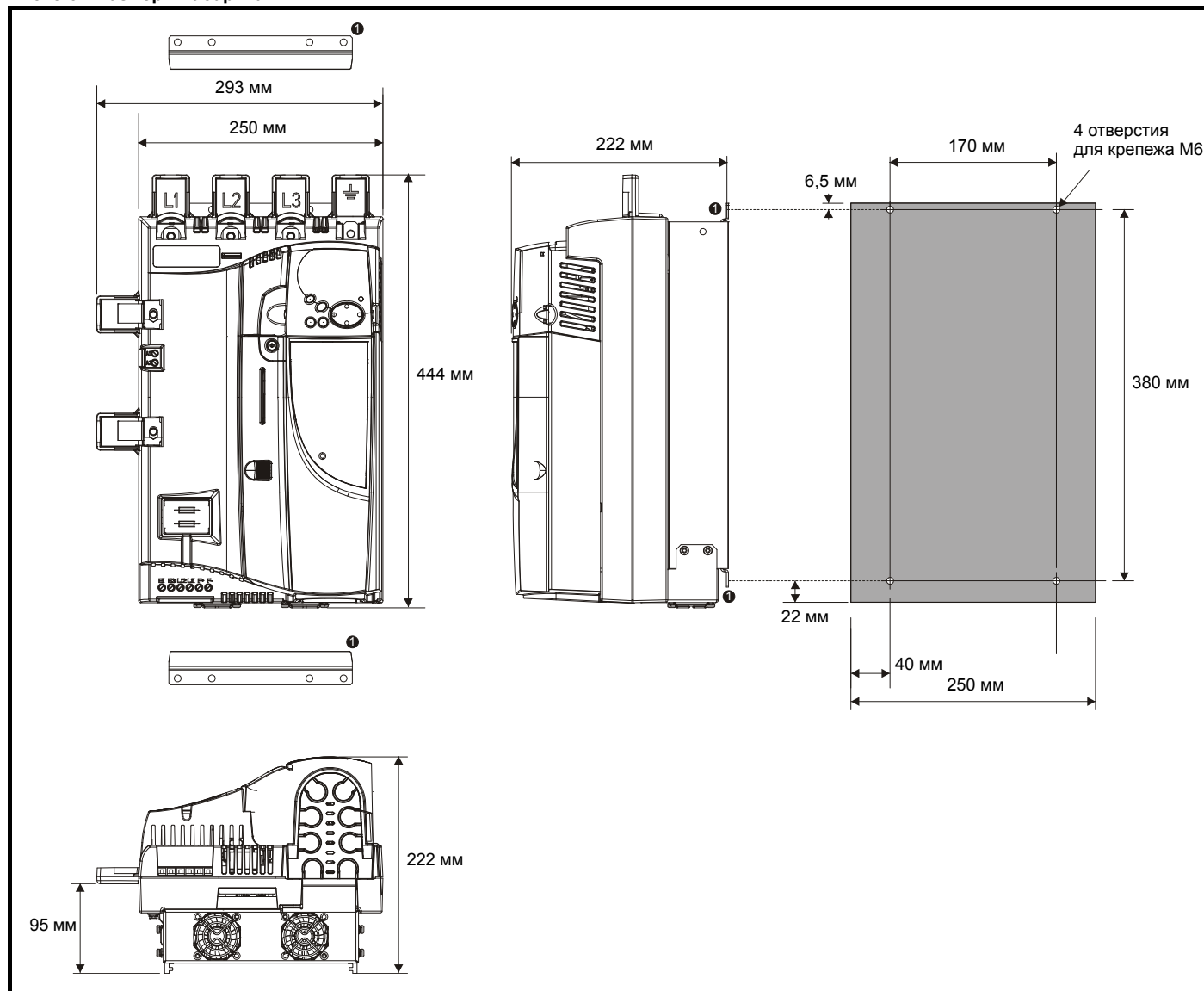
Рис. 3-3 Размеры габарита 1А
