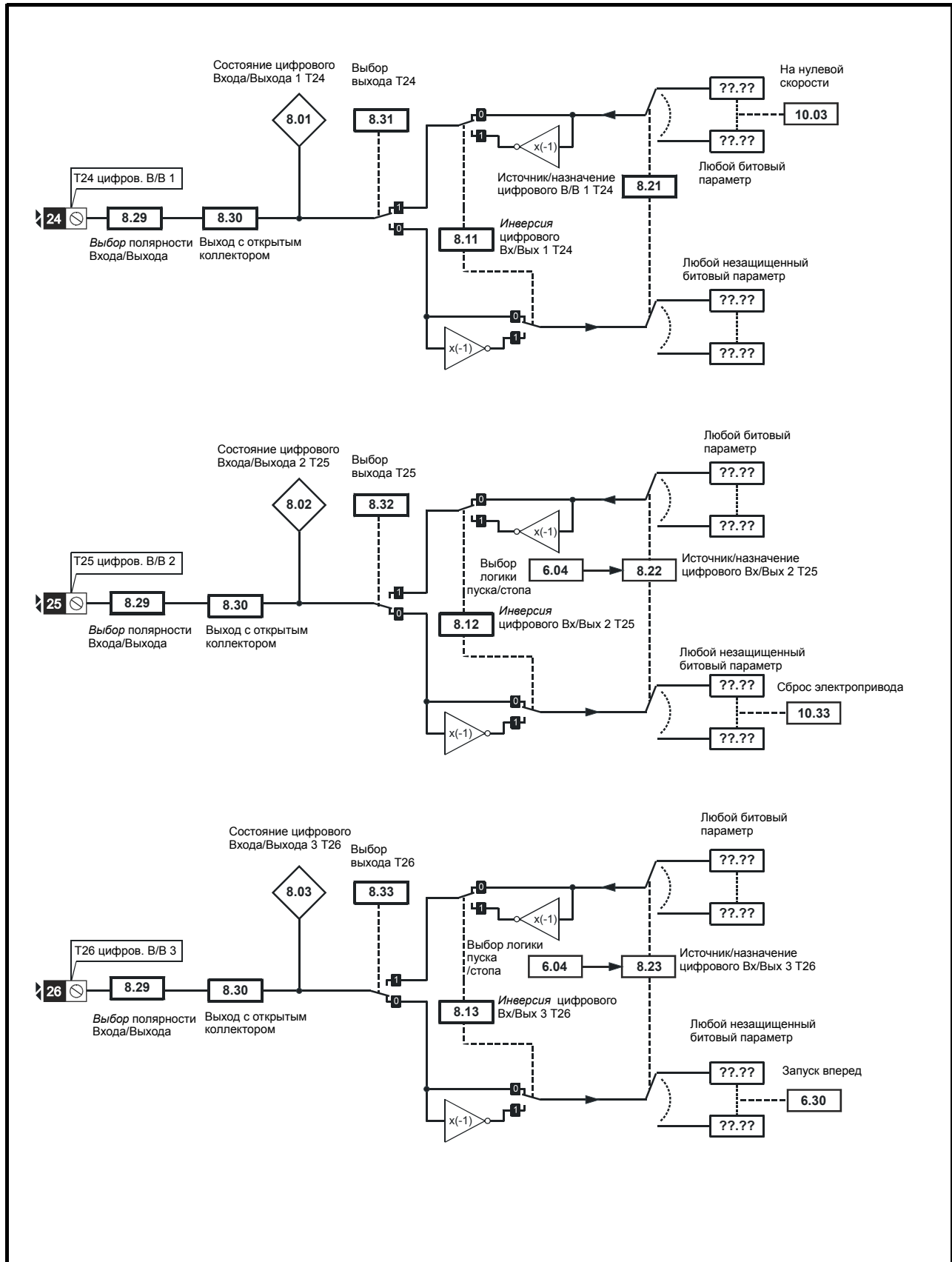
Рис. 8-9 Логическая схема Меню 8
