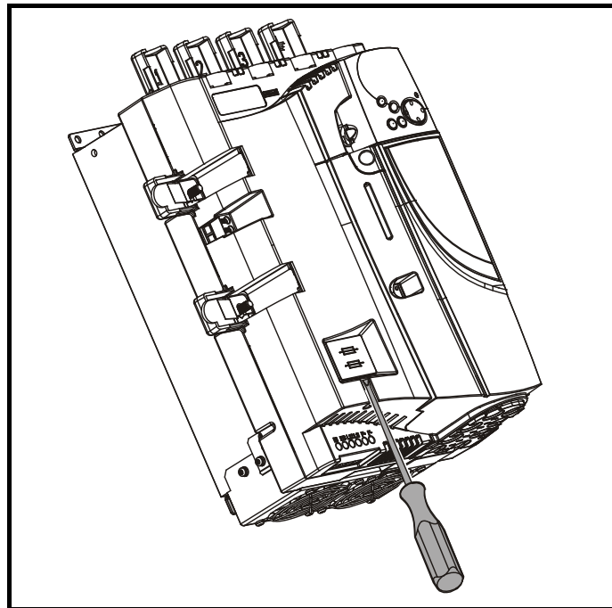
Рис. 4-3 Снятие внутренних предохранителей вспомогательных цепей
