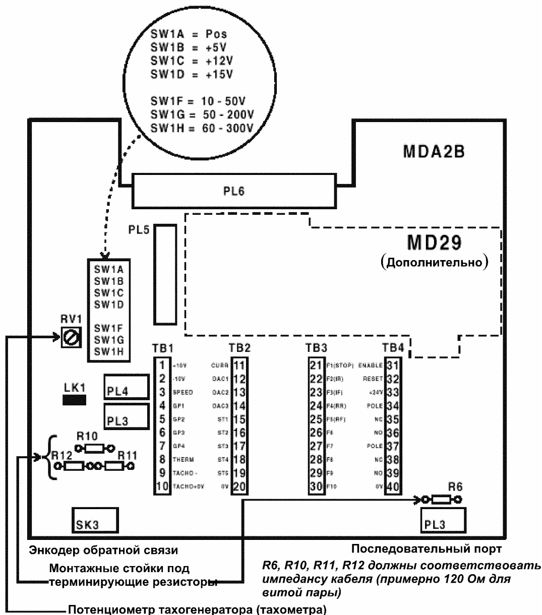
Расположение основных элементов на силовой плате MDA2B выпуска (версии) 2.
