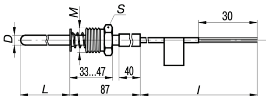
Рисунок А.8 – Конструктивные исполнения 124, 134 и 144
