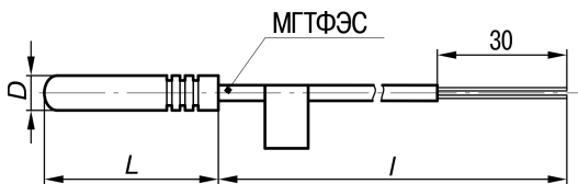
Рисунок А.3 – Конструктивные исполнения 414
