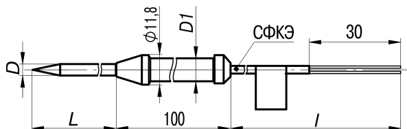
Рисунок А.10 – Конструктивные исполнения 164, 174 и 184
