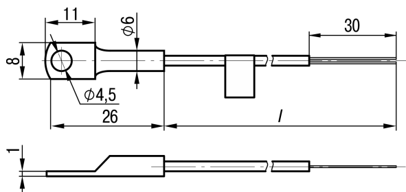
Рисунок А.13 – Конструктивное исполнение 324
