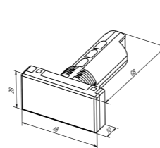
Рисунок 2 – Габаритные размеры корпуса Щ9
