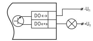
Рисунок 6 – Схема подключения выходного устройства
