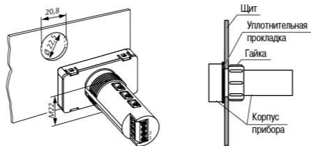
Рисунок 1 – Монтаж прибора щитового крепления
