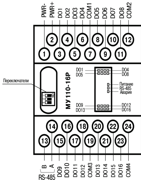
Рисунок Б.1 – Общий чертёж МУ110-16Р и МУ110-16К
