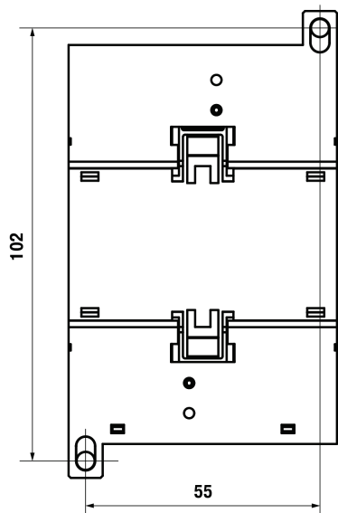
Рисунок А.2 – Установочный чертеж МВ110-224.1ТД
