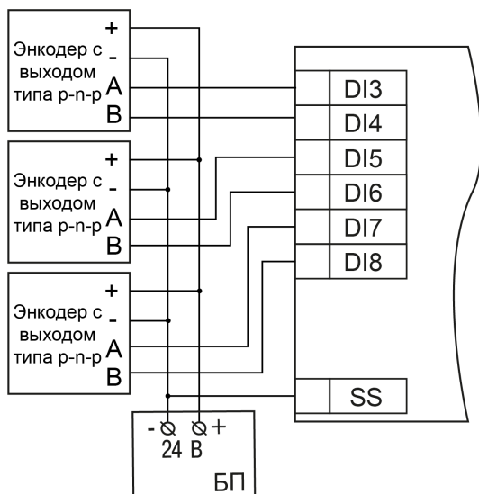
Рисунок 5.8 – Подключение энкодеров типа р-п-р
