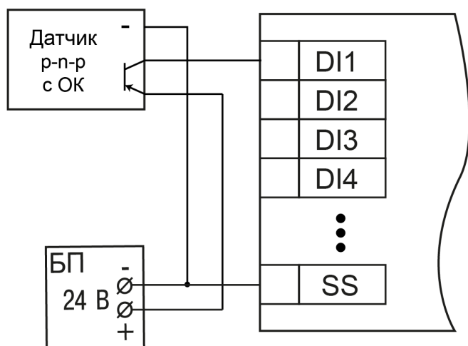
Рисунок 5.6 – Подключение транзисторов р-п-р (только для ОВЕН MB210-202)
