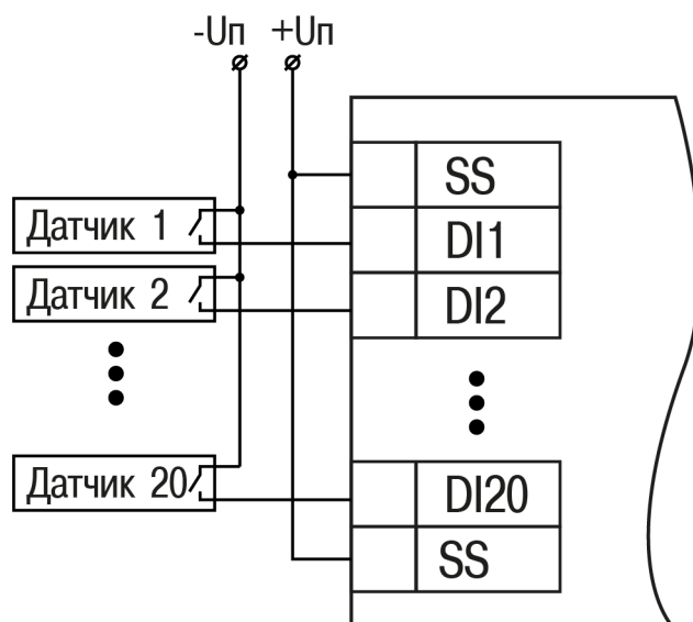
Рисунок 5.4 – Схема подключения к входам DI1–DI20 ОВЕН MB210-202
