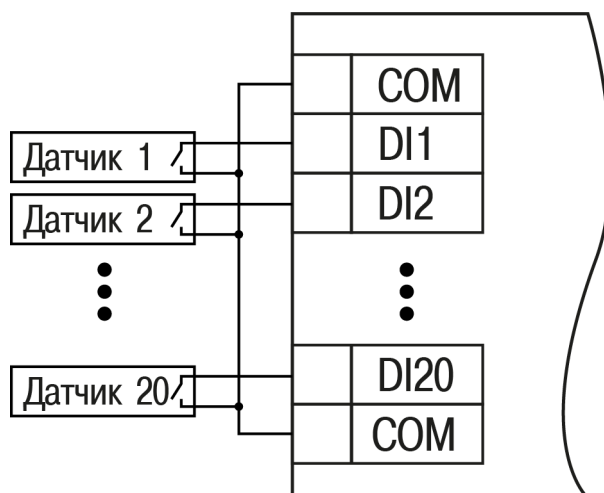
Рисунок 5.5 – Схема подключения к входам DI1–DI20 ОВЕН MB210-204
