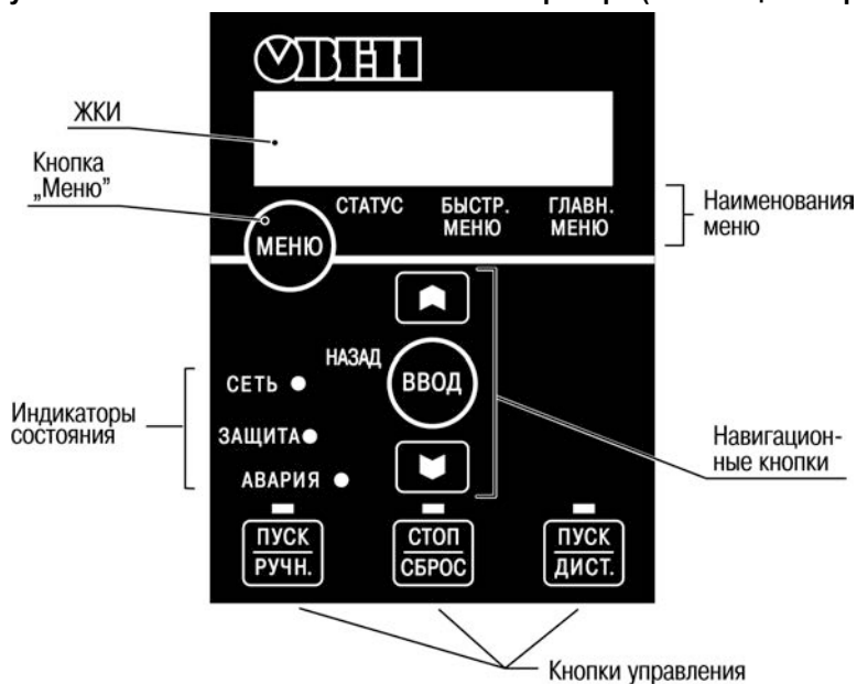
Рисунок 3.3 – ЛПО2 – Локальная панель оператора (без потенциометра)
