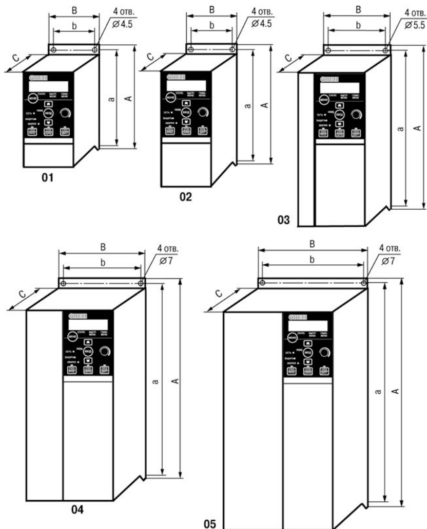
Рисунок А.1 – Габаритные и присоединительные размеры прибора с типоразмерами корпуса 01 – 05. Расшифровка обозначений приведена в таблице А.1.
