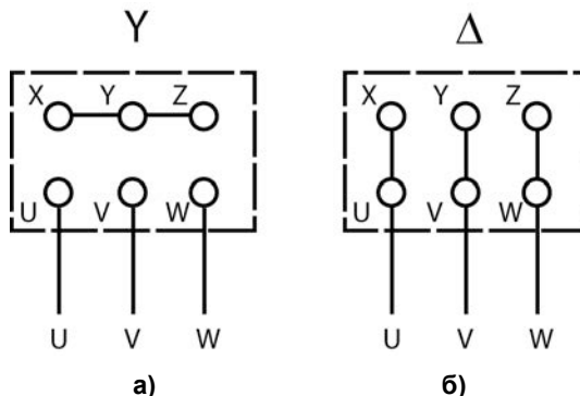
Рисунок 5.3 – Соединения по схемам «звезда» (а) и «треугольник» (б)
