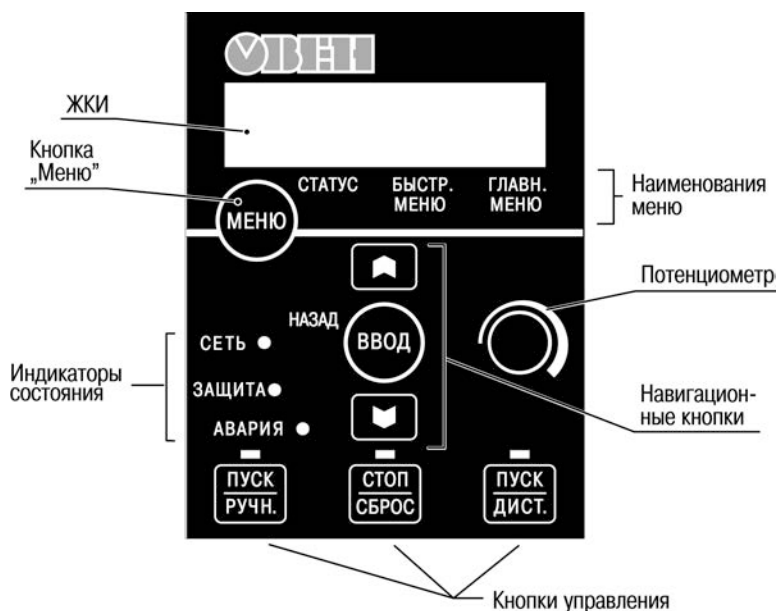
Рисунок 3.2 – ЛПО1 – Локальная панель оператора (с потенциометром)
