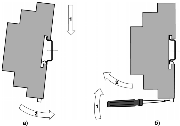
Рисунок 6.1 – Монтаж контроллера на DIN-рейку
