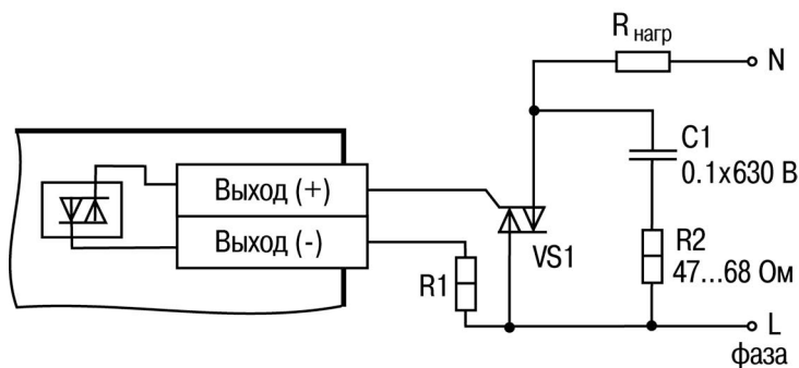
Рисунок Б.12 – Схема подключения нагрузки к ВЭ типа «С»
