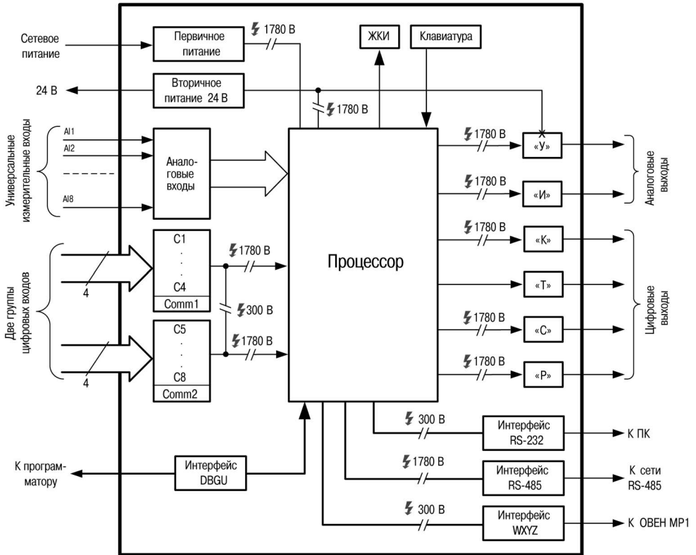
Рисунок 3.2 – Функциональная схема контроллера
