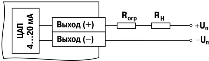
Рисунок 3.3 – Схема подключения нагрузки к ВУ типа «И»
