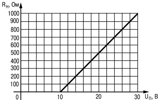
Рисунок 3.4 – График зависимости R_н(U_п)
