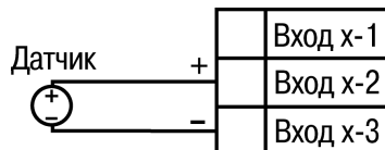
Рисунок Б.5 – Подключение активного датчика с выходом в виде напряжения 0...1 В
