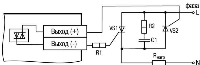
Рисунок Б.13 – Схема подключения нагрузки к ВЭ типа «С» двух тиристор, подключенных встречно-параллельно (R2=47... 68 Ом, C1=0.1мкф×630 В)
