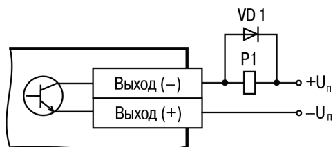
Рисунок Б.11 – Схема подключения нагрузки к ВЭ типа «К» (диод VD1 должен быть рассчитан на напряжение 100 В и ток 1 А)
