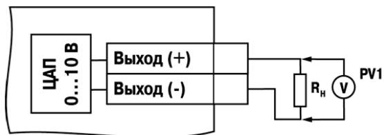
Рисунок Б.8 – Схема подключения нагрузки к ВЭ типа «У». R_H > 2 \text{ кОм}
