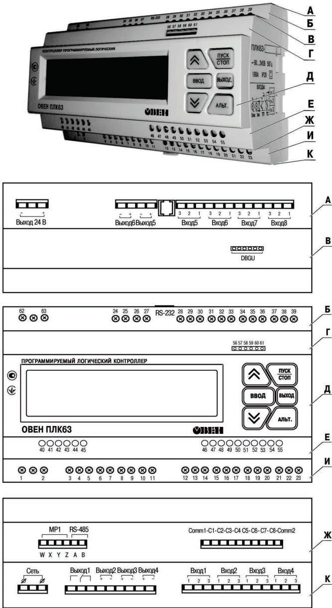
Рисунок 3.1 – Разъемные соединения, элементы индикации и управления контроллера
