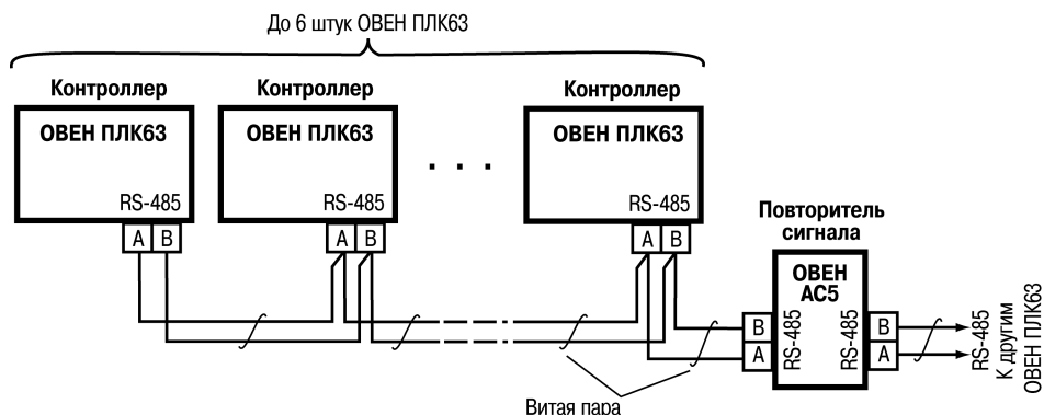
Рисунок 6.3 – Пример схемы подключений в сеть более 6-ти ОВЕН ПЛК63 (ОВЕН АС5 – повторитель сигнала)
