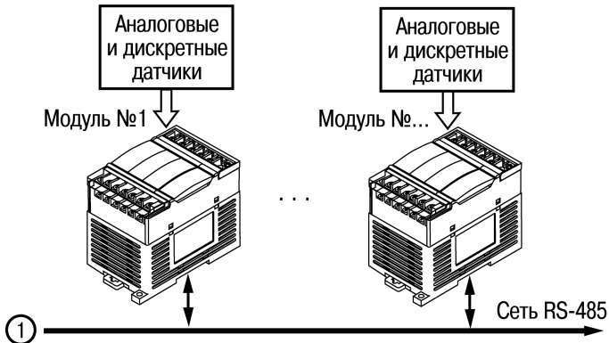
Рисунок 6.4 – Пример структуры соединений при использовании ПЛК в системе
