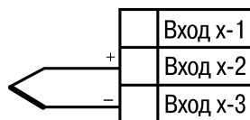
Рисунок Б.7 – Схема подключения преобразователя термоэлектрического (термопары)
