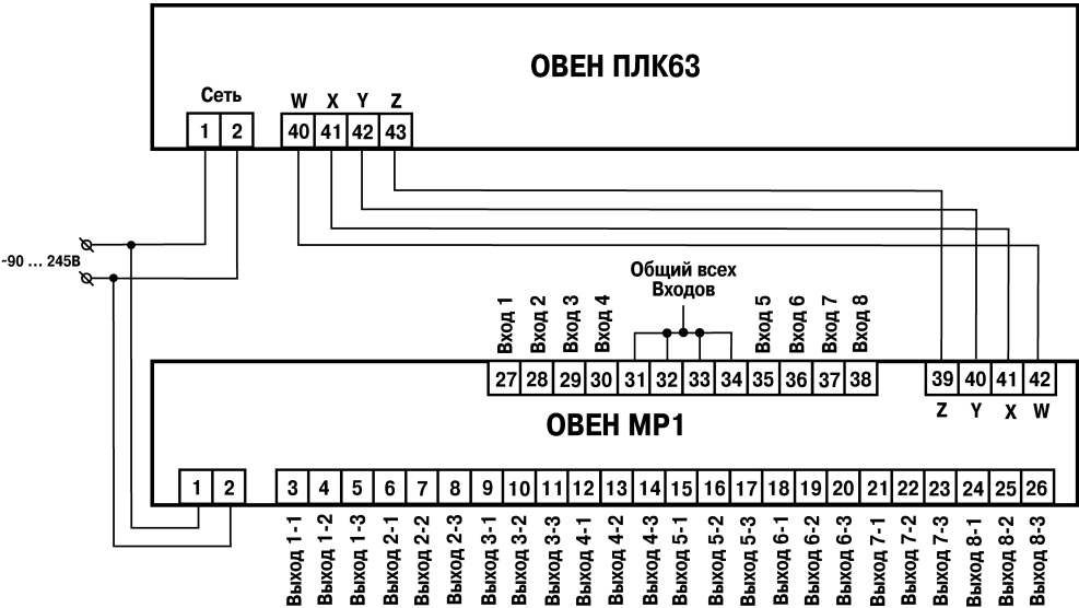
Рисунок Б.16 – Схема подключения модуля ОВЕН MP1 к контроллеру
