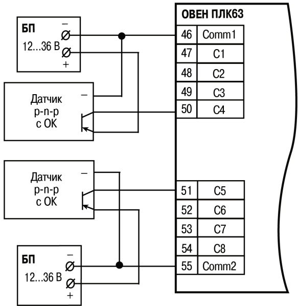
Рисунок Б.2 – Схема подключения р-п-р датчиков
