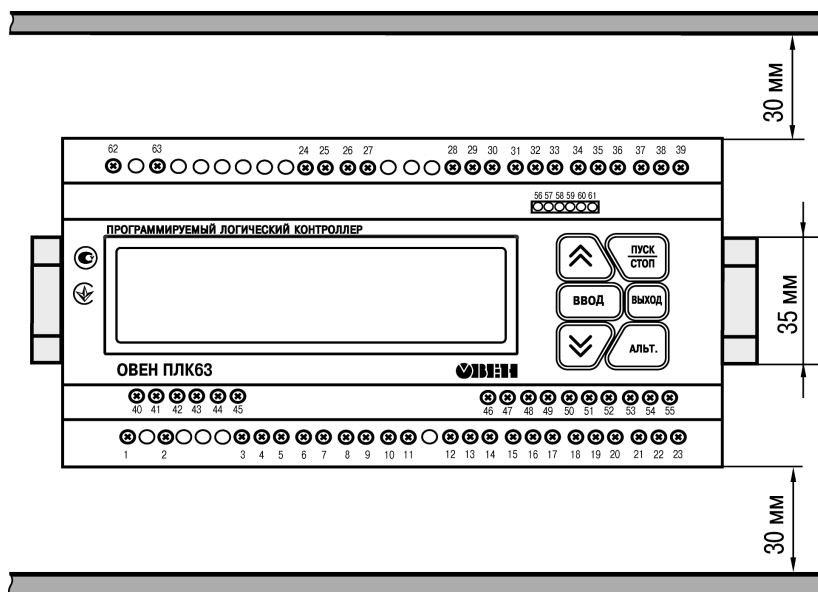
Рисунок А.3 – Расстояние до стенок корпуса контроллера при монтаже для обеспечения вентиляции
