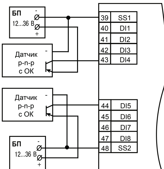
Рисунок Б.2 – Схема подключения р-н-р датчиков
