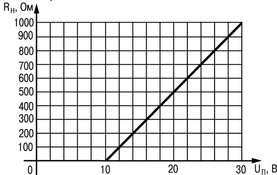
Рисунок 3.4 – График зависимости R_n (U_n)
