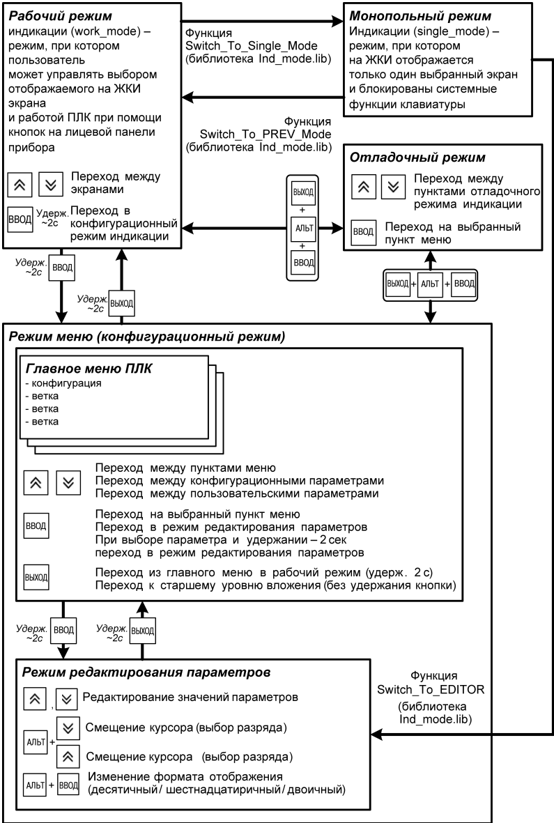
Рисунок 7.1 – Диаграмма переходов между режимами индикации контроллера
