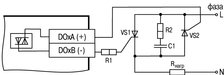
Рисунок Б.13 – Схема подключения нагрузки к ВЭ типа «С» двух тиристоров, подключенных встречно-параллельно ( R_2=47... 68 \text{ Ом} , C_1=0.1\text{мкф}\times 630 \text{ В} )
