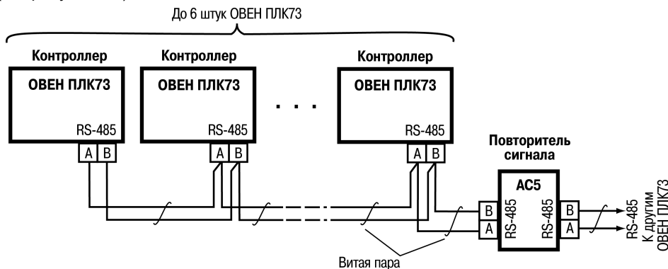
Рисунок 6.3 – Пример схемы подключений в сеть более 6-ти ОБЕН ПЛК73 (АС5 – повторитель сигнала разработки ОБЕН)
