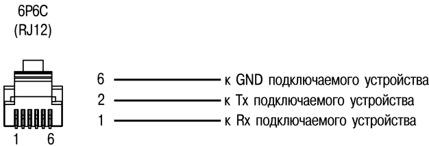
Рисунок В.3 – Схема кабеля для подключения контроллера к порту RS-232
