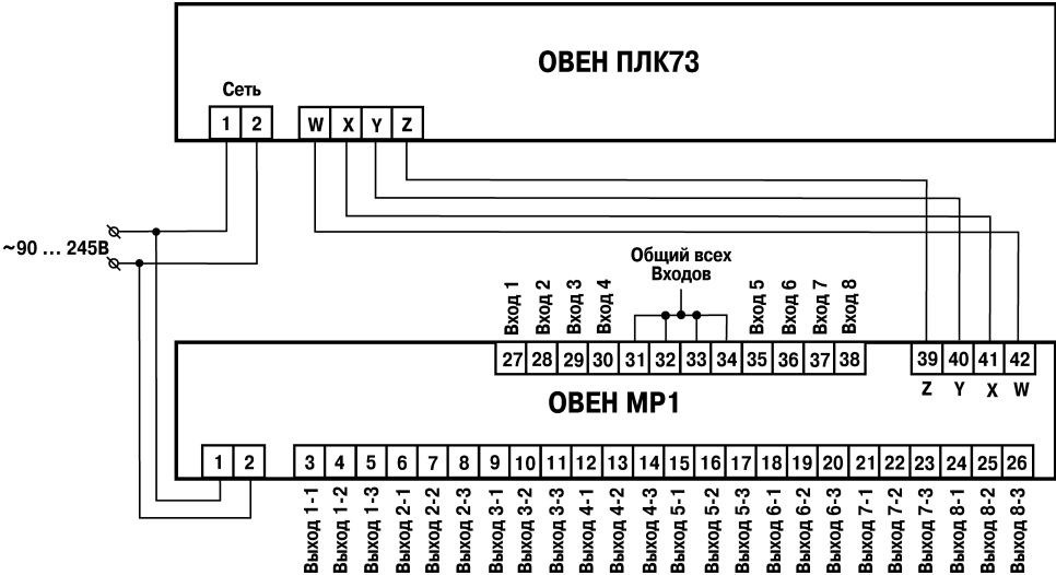
Рисунок Б.15 – Схема подключения модуля ОВЕН МР1 к ОВЕН ПЛК73
