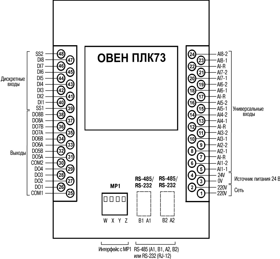
Рисунок Б.16 – Схема расположения и назначения клемм контроллера (вид на заднюю стенку корпуса)
