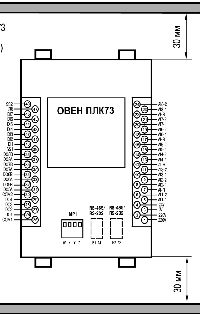
Рисунок А.2 – Расстояние до стенок корпуса контроллера при монтаже для обеспечения вентиляции
