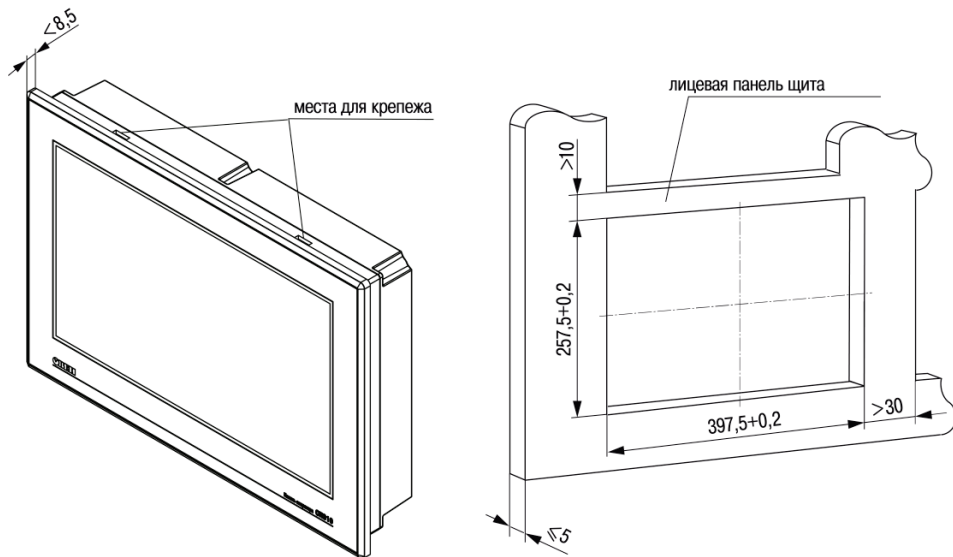
Рисунок А.6 – Установочные размеры СП315
