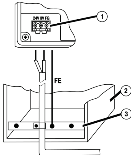
Рисунок Б.1 – Подключение выравнивающих потенциалы защитного заземления
