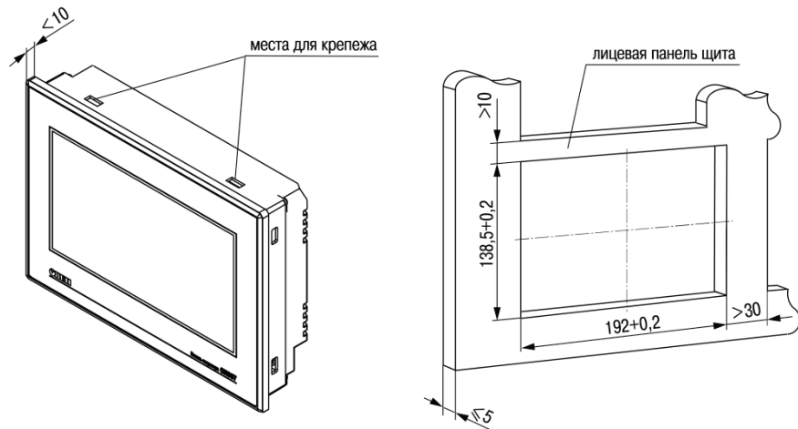
Рисунок А.4 – Установочные размеры СП307
