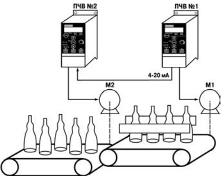
Рисунок 4.14 – Схема установки
