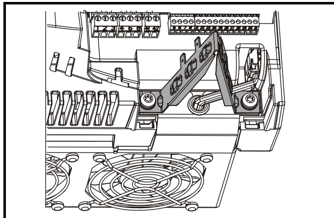
Рис. 4-18 Заземление экрана сигнального кабеля с помощью скобы заземления
