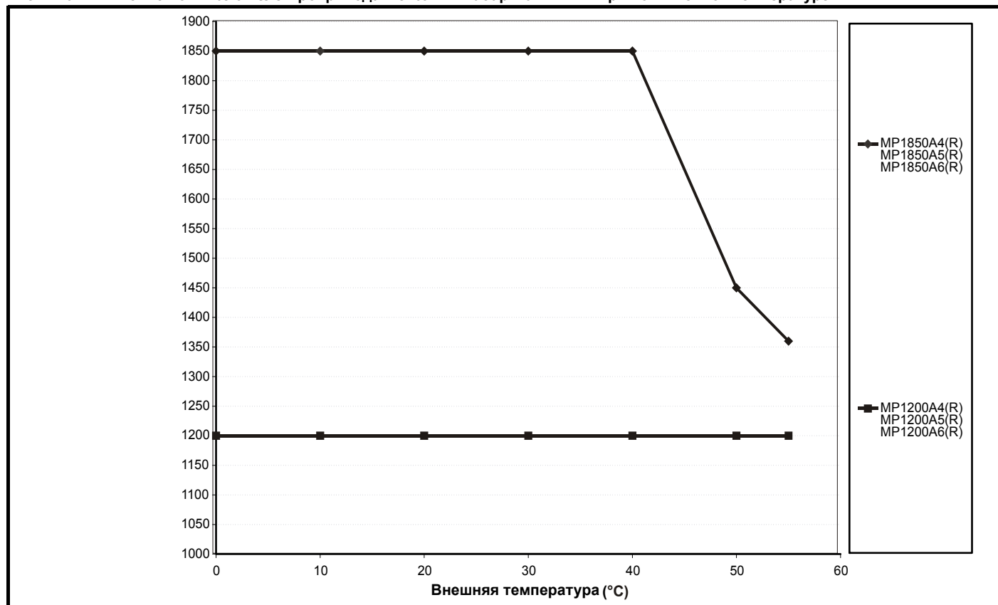
Рис. 12-6 Снижение номиналов электропривода Mentor MP габарита 2C и 2D при повышенной температуре
