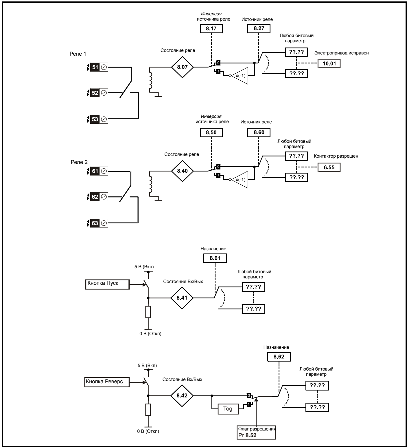
Рис. 11-11 Логическая схема Меню 8 (продолжение)
