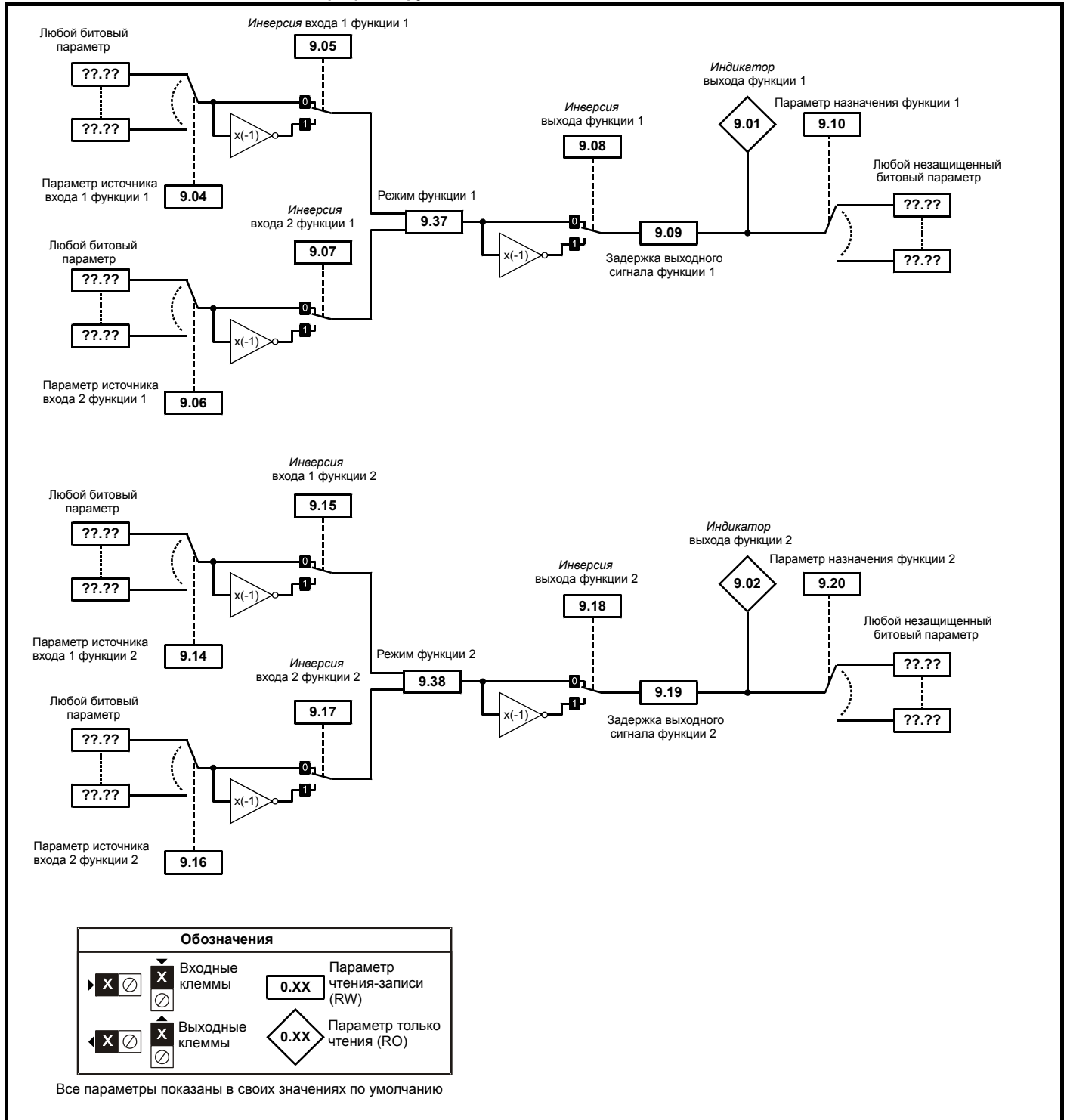
Рис. 11-12 Логическая схема Меню 9: Программируемая логика
