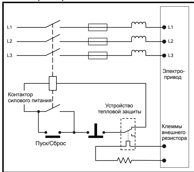
Рис. 4-13 Схема защиты внешнего ограничительного резистора
