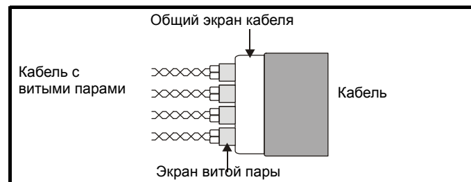
Рис. 4-21 Кабель обратной связи, витая пара
