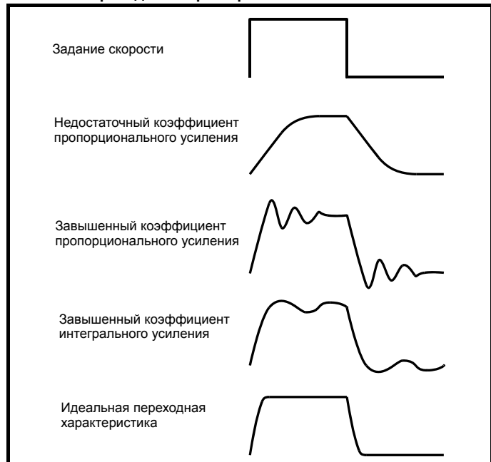
Рис. 8-1 Переходные характеристики
