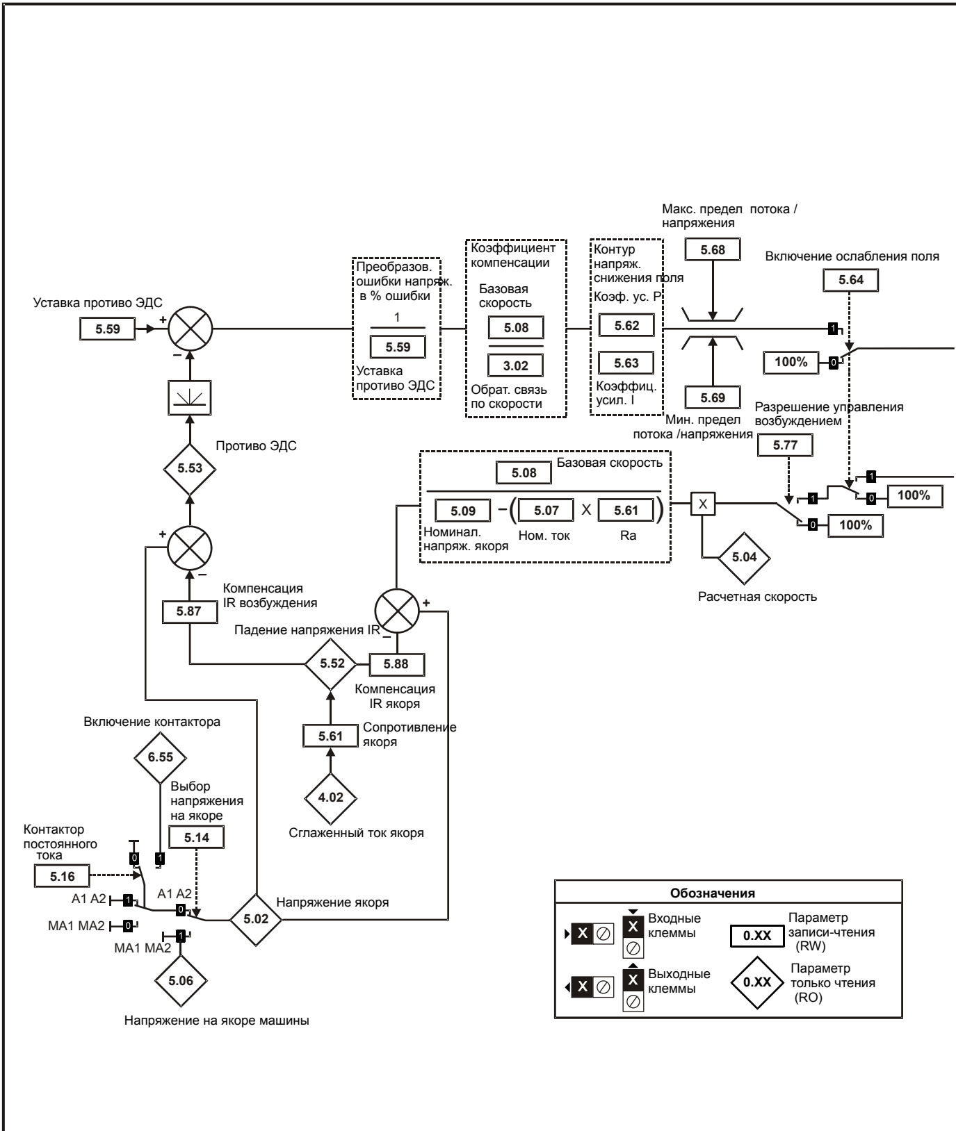
Рис. 11-5 Меню 5 - логическая схема управления якорем
