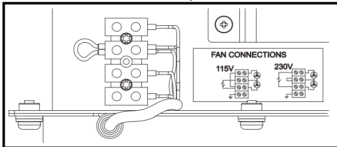
Рис. 4-19 Подключение вентилятора
