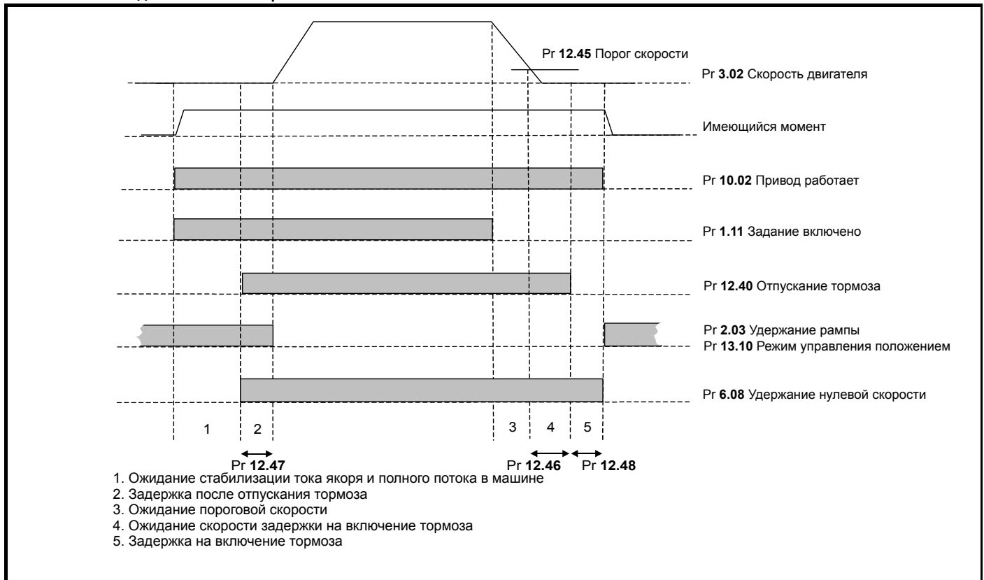
Рис. 11-17 Последовательность торможения
