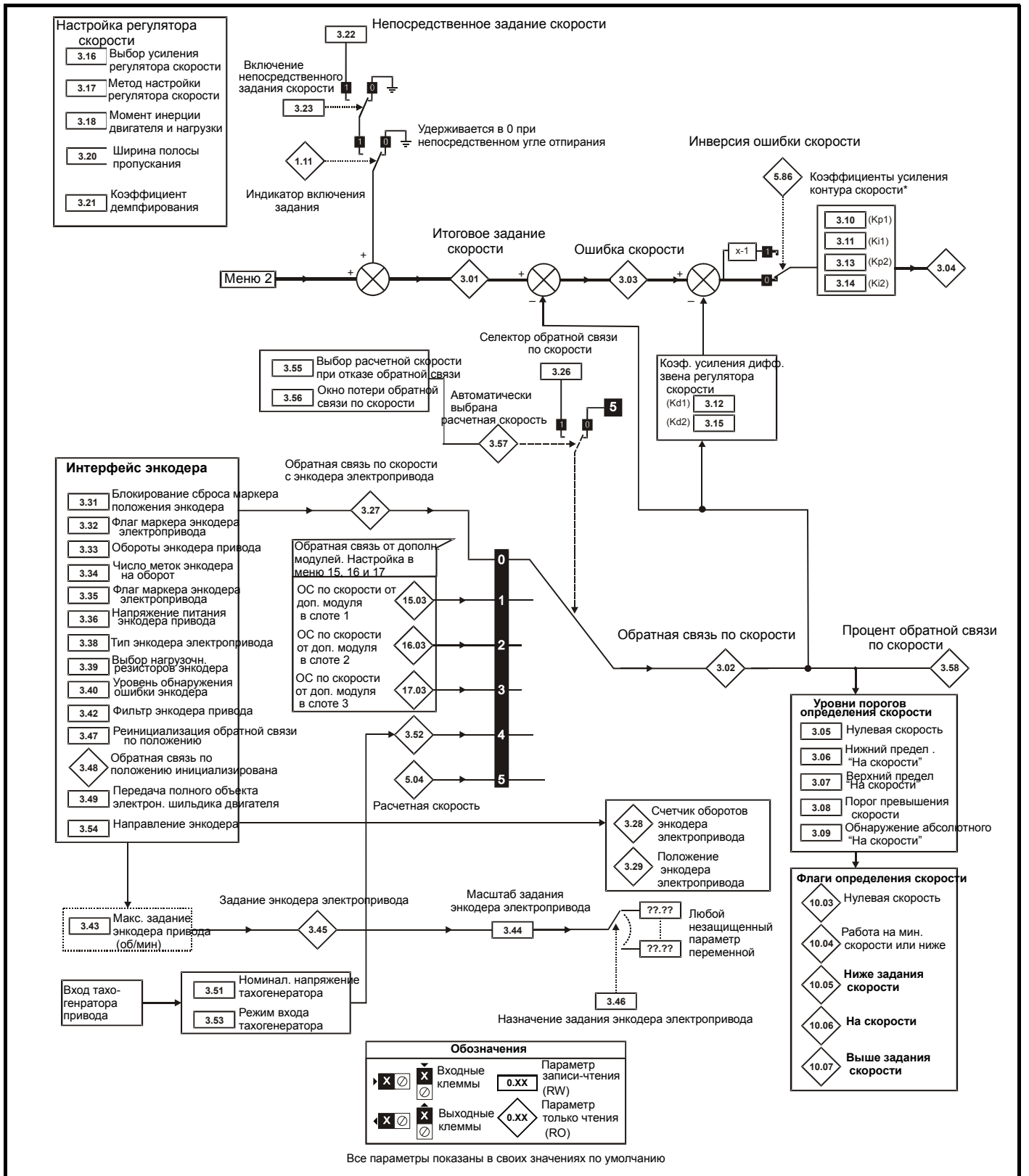
Рис. 11-3 Логическая схема Меню 3
