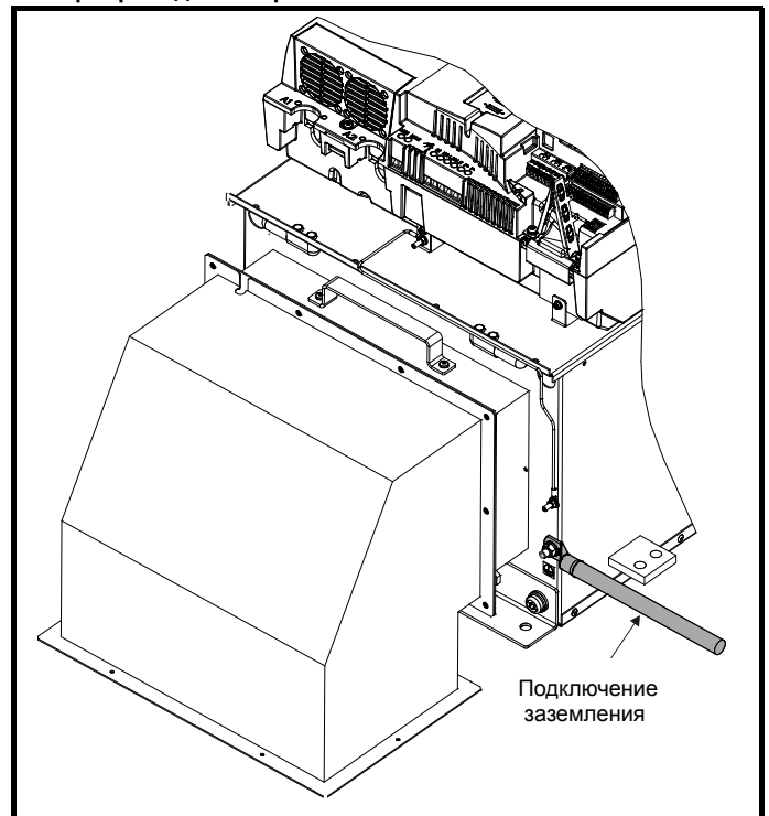
Рис. 4-5 Расположение подключения заземления на электроприводах габарита 2C / 2D
