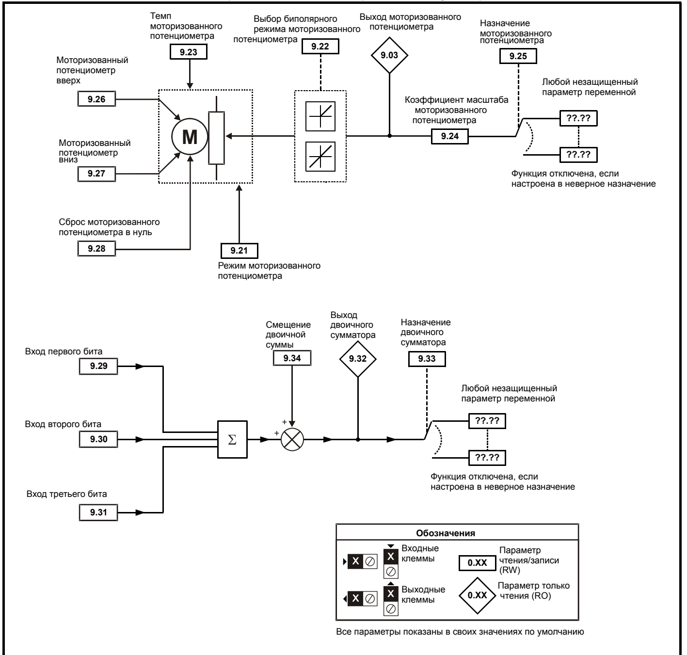
Рис. 11-13 Логическая схема Меню 9: Моторизованный потенциометр и двоичный сумматор
