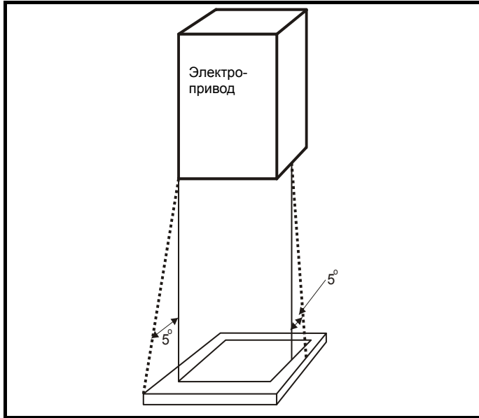
Рис. 3-1 Компоновка дна огнестойкого корпуса
