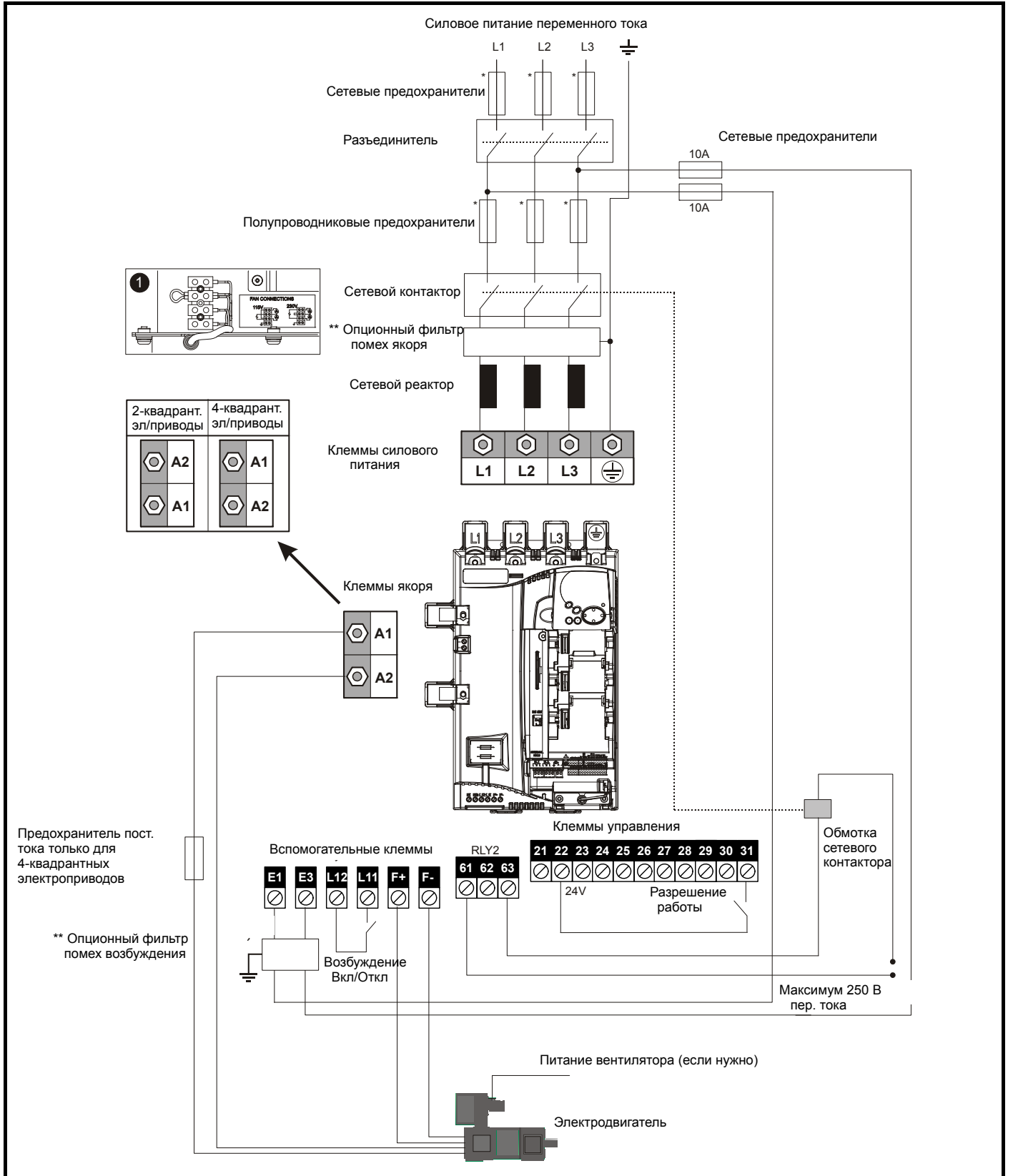
Рис. 4-1 Силовые подключения для электропривода 480 В
