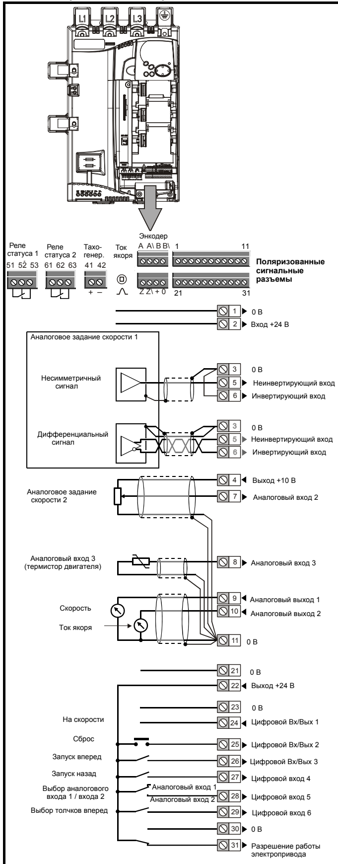
Рис. 4-20 Функции клемм по умолчанию
