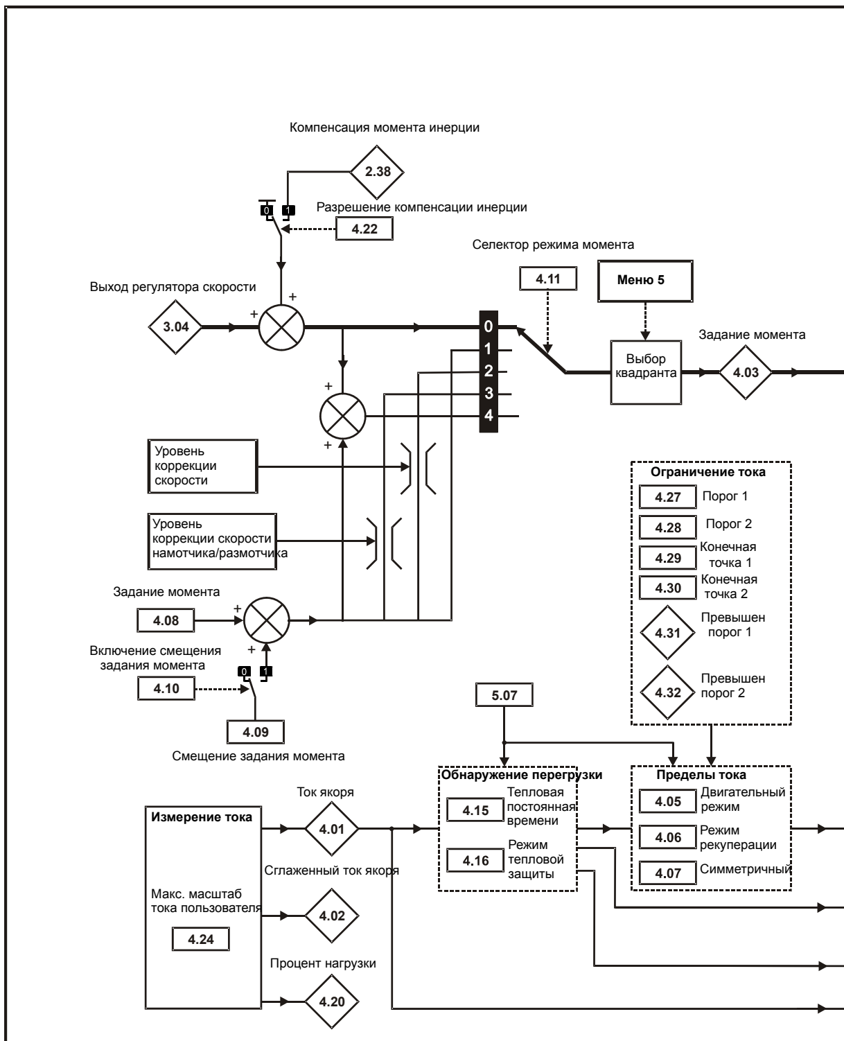
Рис. 11-4 Логическая схема Меню 4
