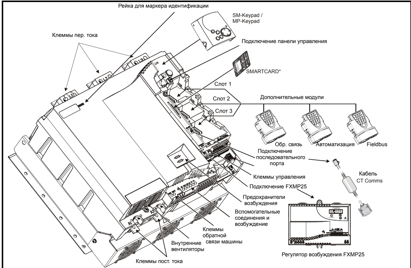
Рис. 2-5 Общий вид и опции электропривода габарита 2
