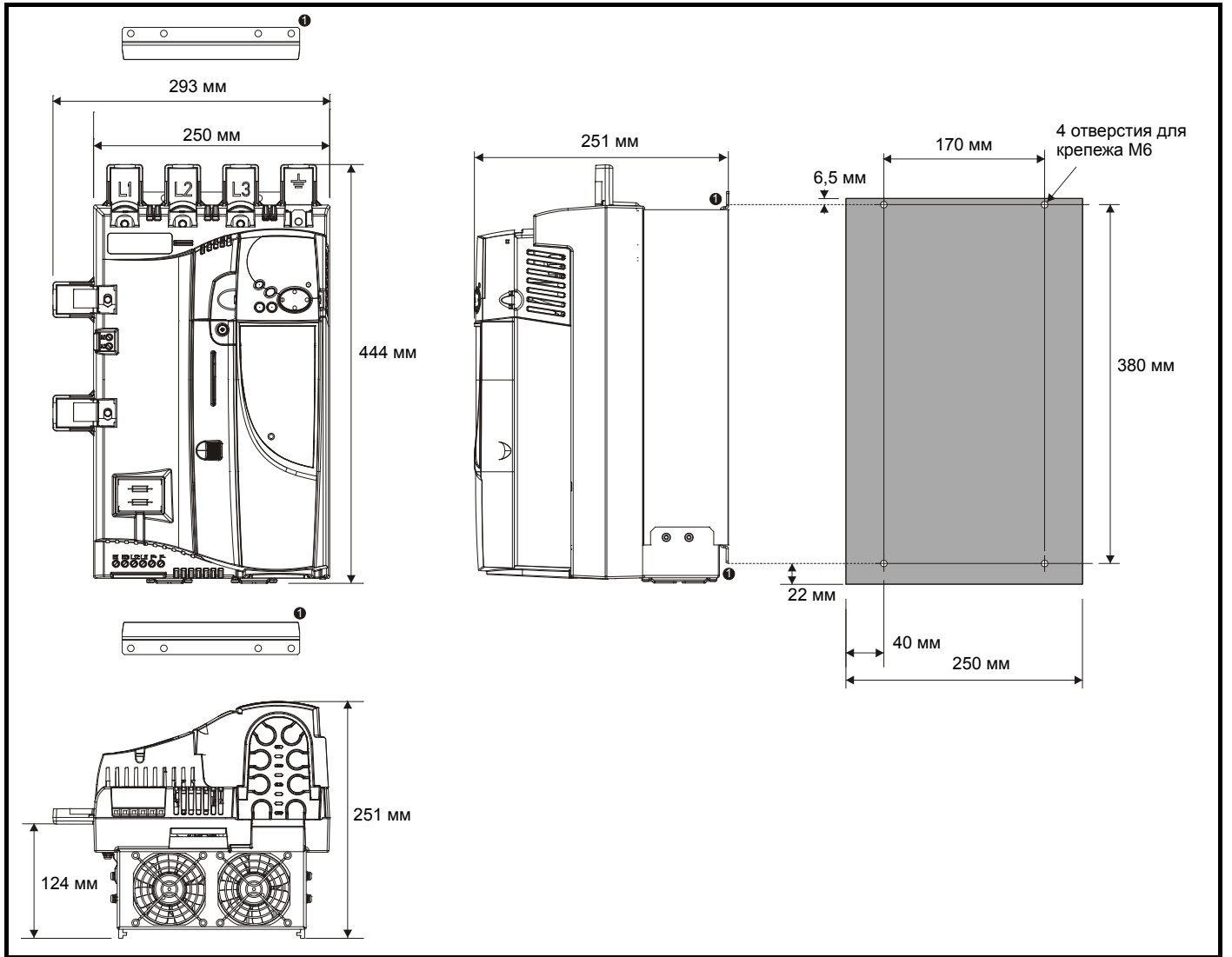
Рис. 3-8 Размеры габарита 1В
