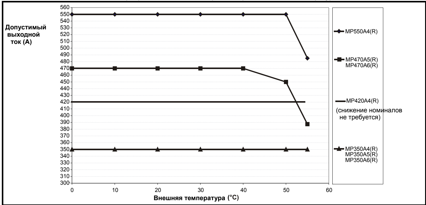
Рис. 12-5 Снижение номиналов электропривода Mentor MP габарита 2B при повышенной температуре
