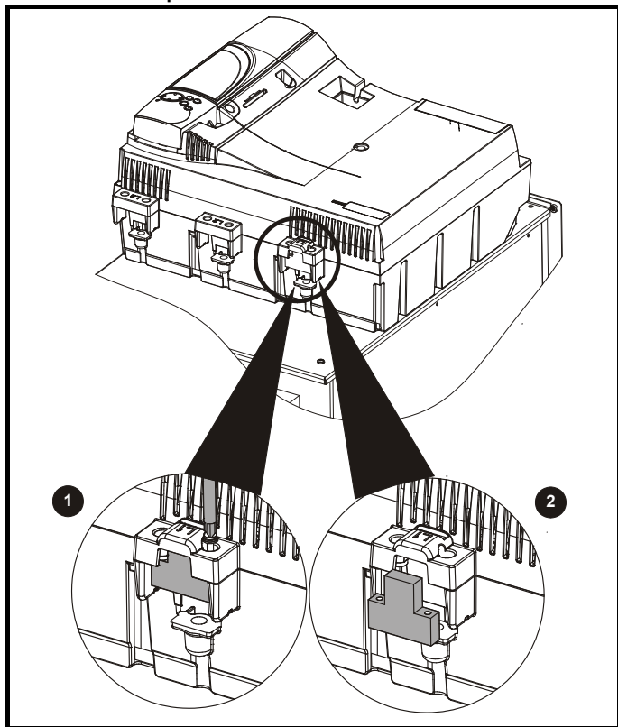
Рис. 4-12 Снятие крышки клемм подавления выбросов на габаритах 2C и 2D
