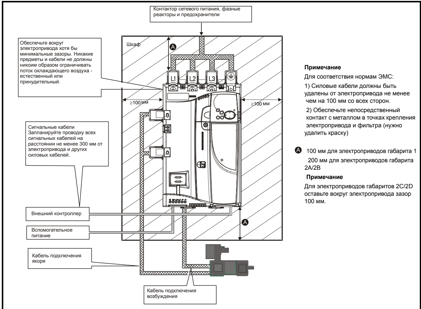
Рис. 3-21 Компоновка шкафа
