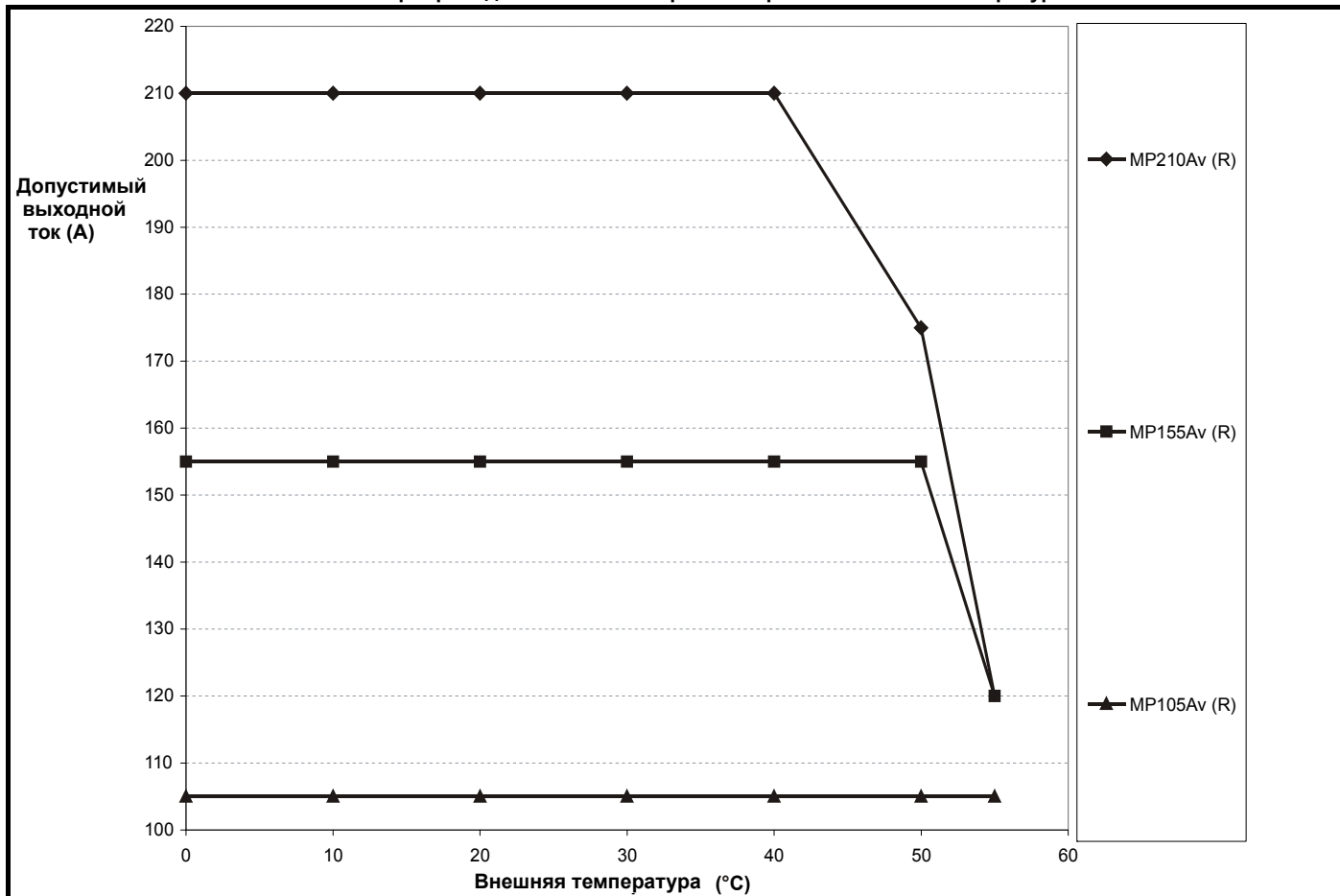
Рис. 12-3 Снижение номиналов электропривода Mentor MP габарита 1B при повышенной температуре
