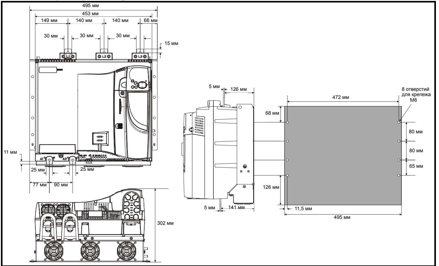
Рис. 3-12 Размеры габарита 2B без установленных чехлов клемм
