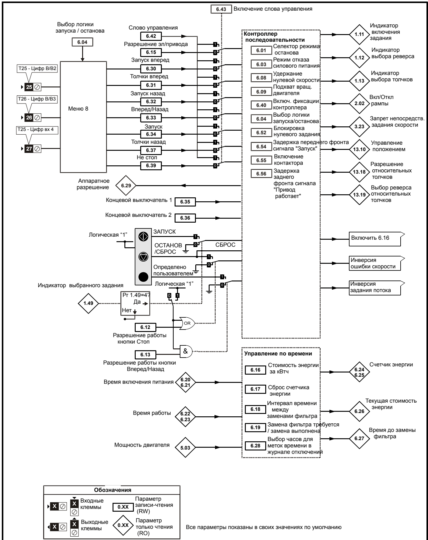
Рис. 11-7 Логическая схема Меню 6
