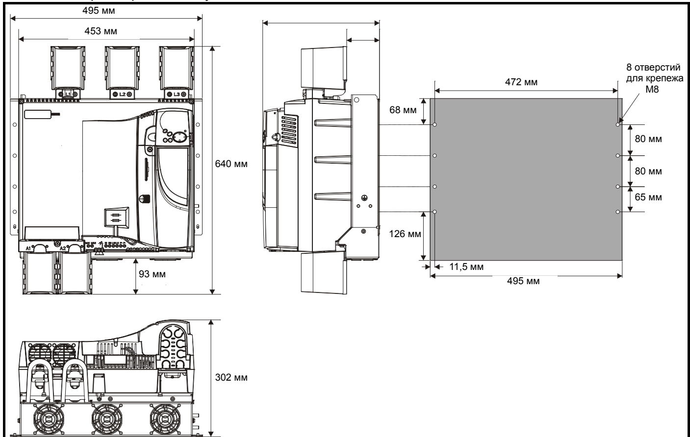
Рис. 3-10 Размеры габарита 2А / 2В с установленными чехлами клемм
