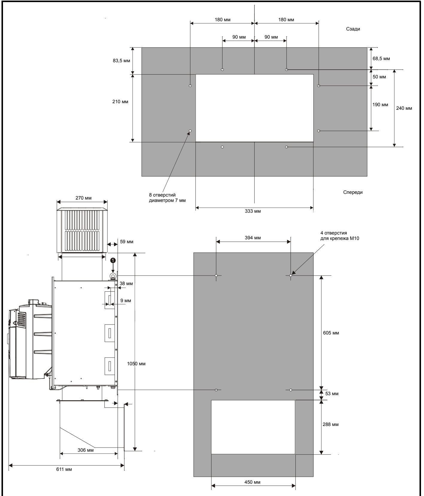
Рис. 3-14 Задняя пластина и вид монтажа габарита 2С
