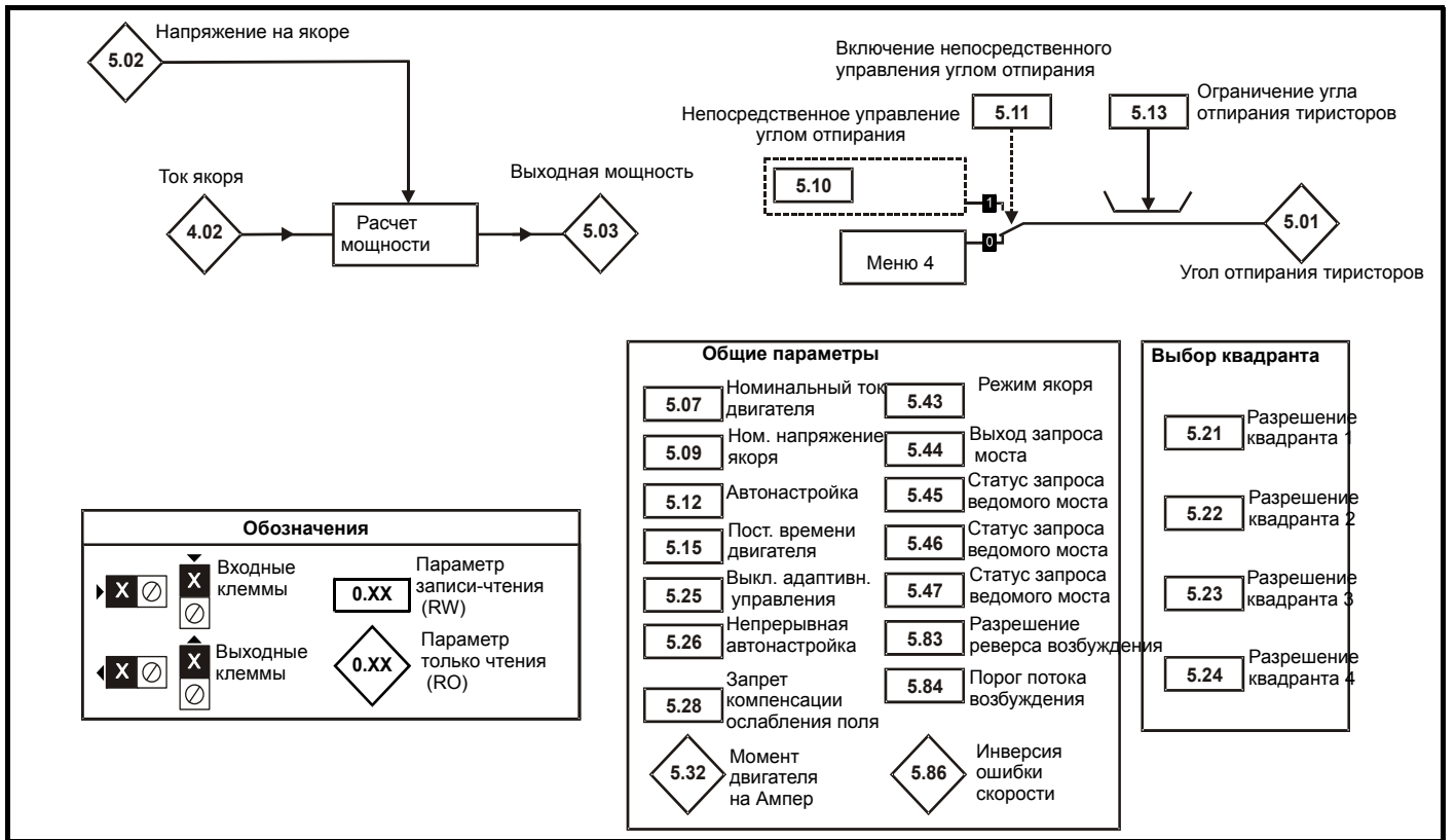
Рис. 11-6 Меню 5 - логическая схема управления якорем
