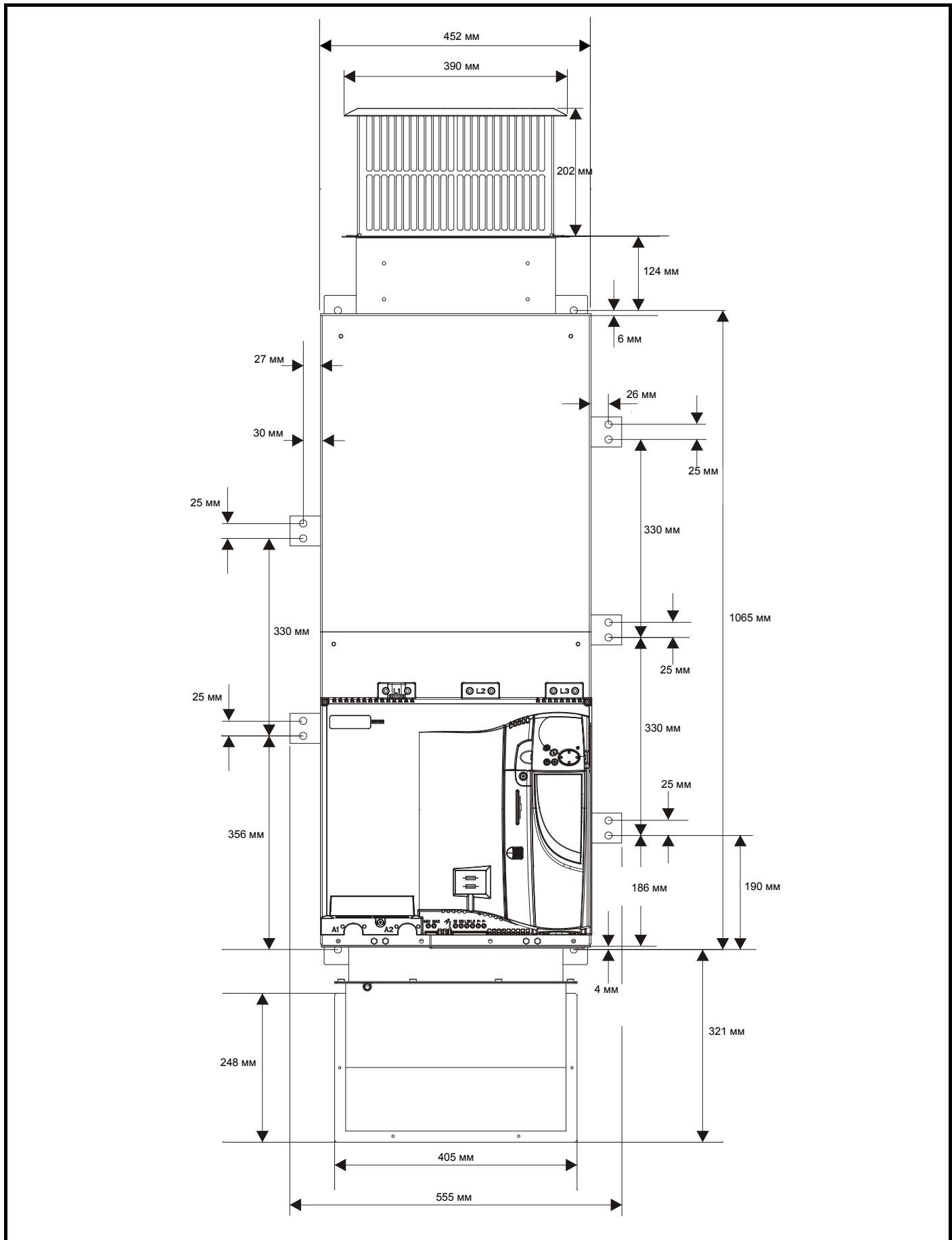
Рис. 3-15 Вид спереди и монтажные размеры габарита 2D
