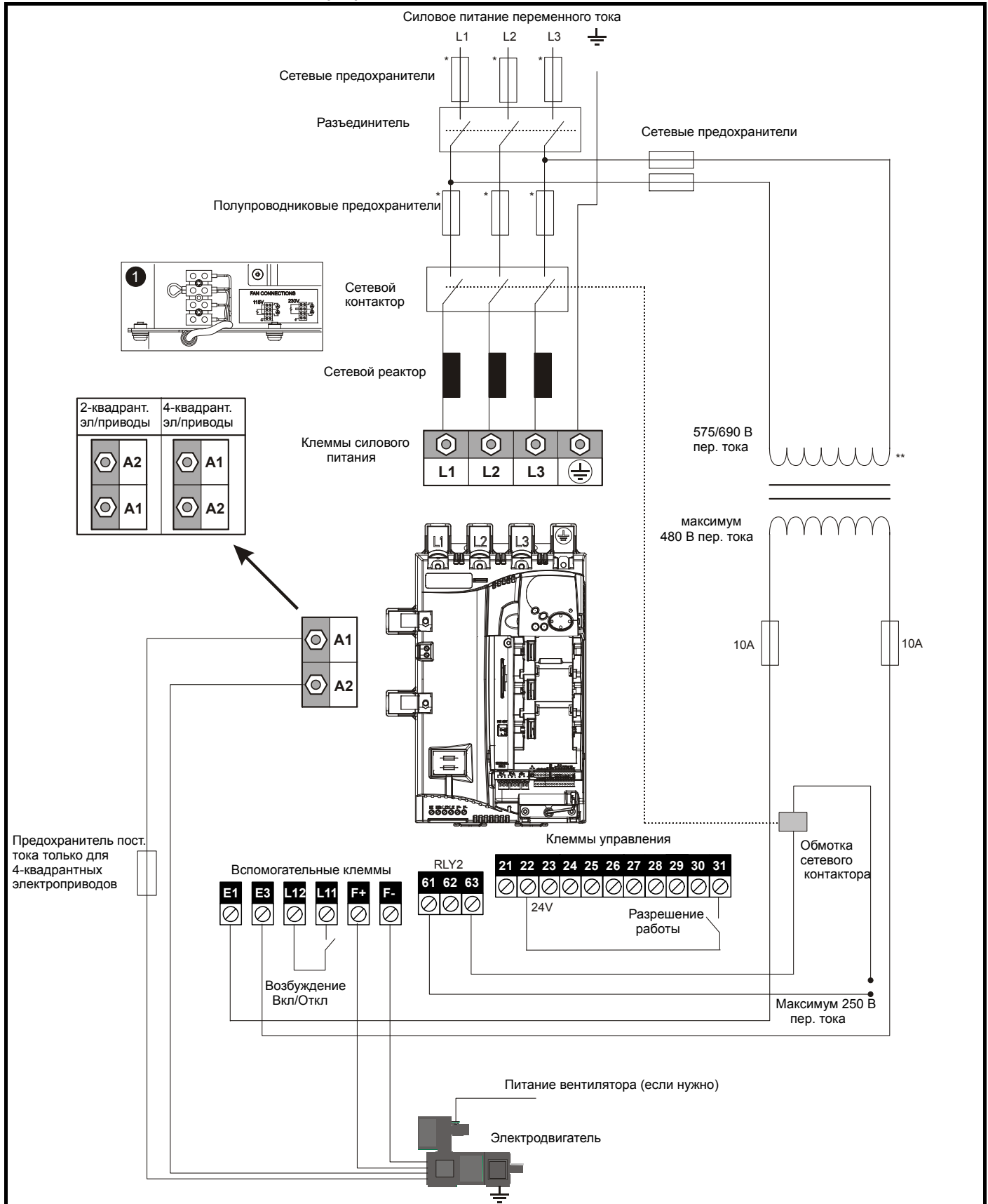
Рис. 4-2 Силовые подключения для электроприводов 575 / 600 / 690 В
