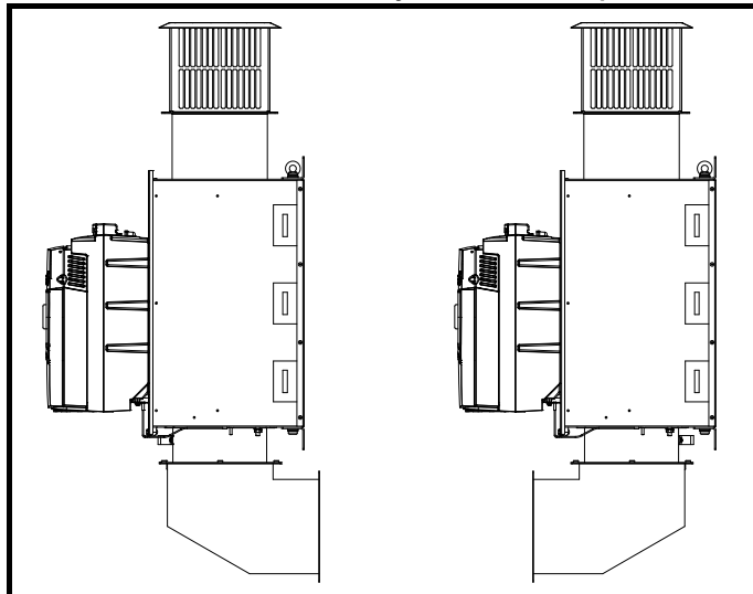
Рис. 3-17 Методы монтажа воздуховода для габарита 2С / 2D
