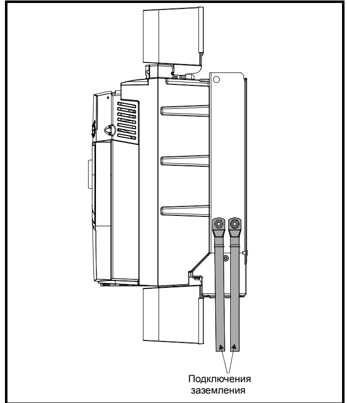
Рис. 4-5 Расположение подключения заземления на электроприводах габарита 2C / 2D
