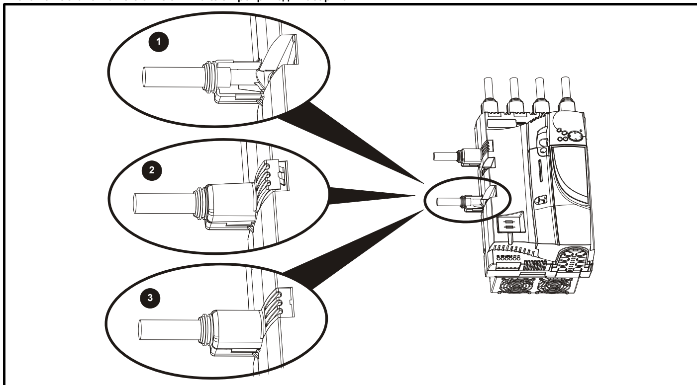
Рис. 3-18 Установка чехлов клемм на электроприводы габарита 1
