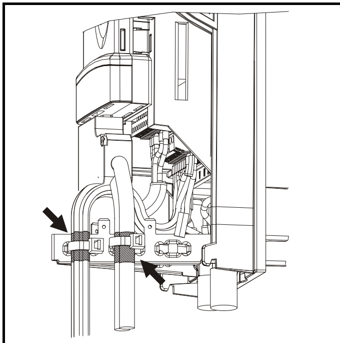
Рис. 4-18 Заземление экрана сигнального кабеля с помощью скобы заземления
