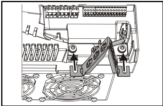
Рис. 4-17 Установка заземляющей скобы
