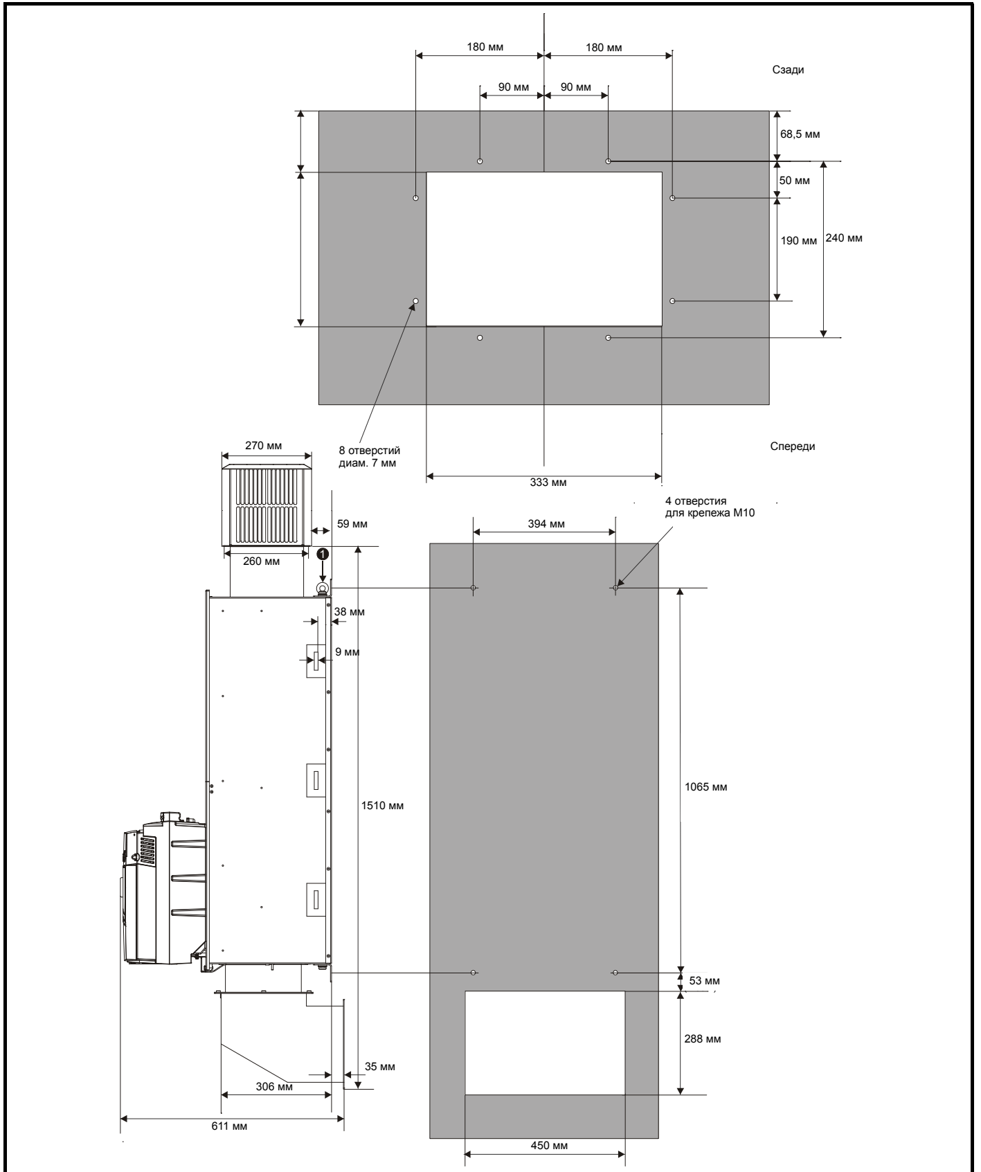
Рис. 3-16 Задняя пластина и вид монтажа габарита 2D
