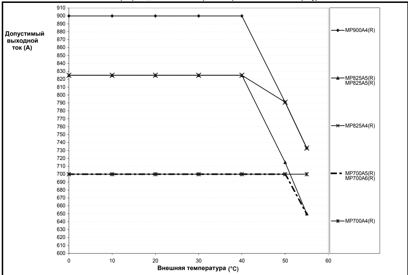
Рис. 12-5 Снижение номиналов электропривода Mentor MP габарита 2B при повышенной температуре
