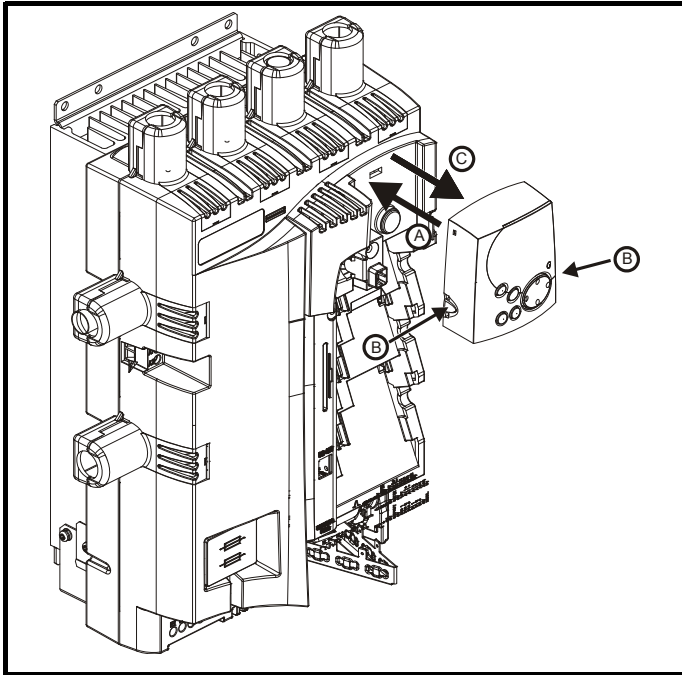
Рис. 3-6 Снятие и установка панели управления
