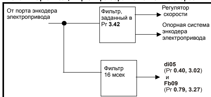
Рис. 6-1 Организация фильтра обратной связи по скорости
