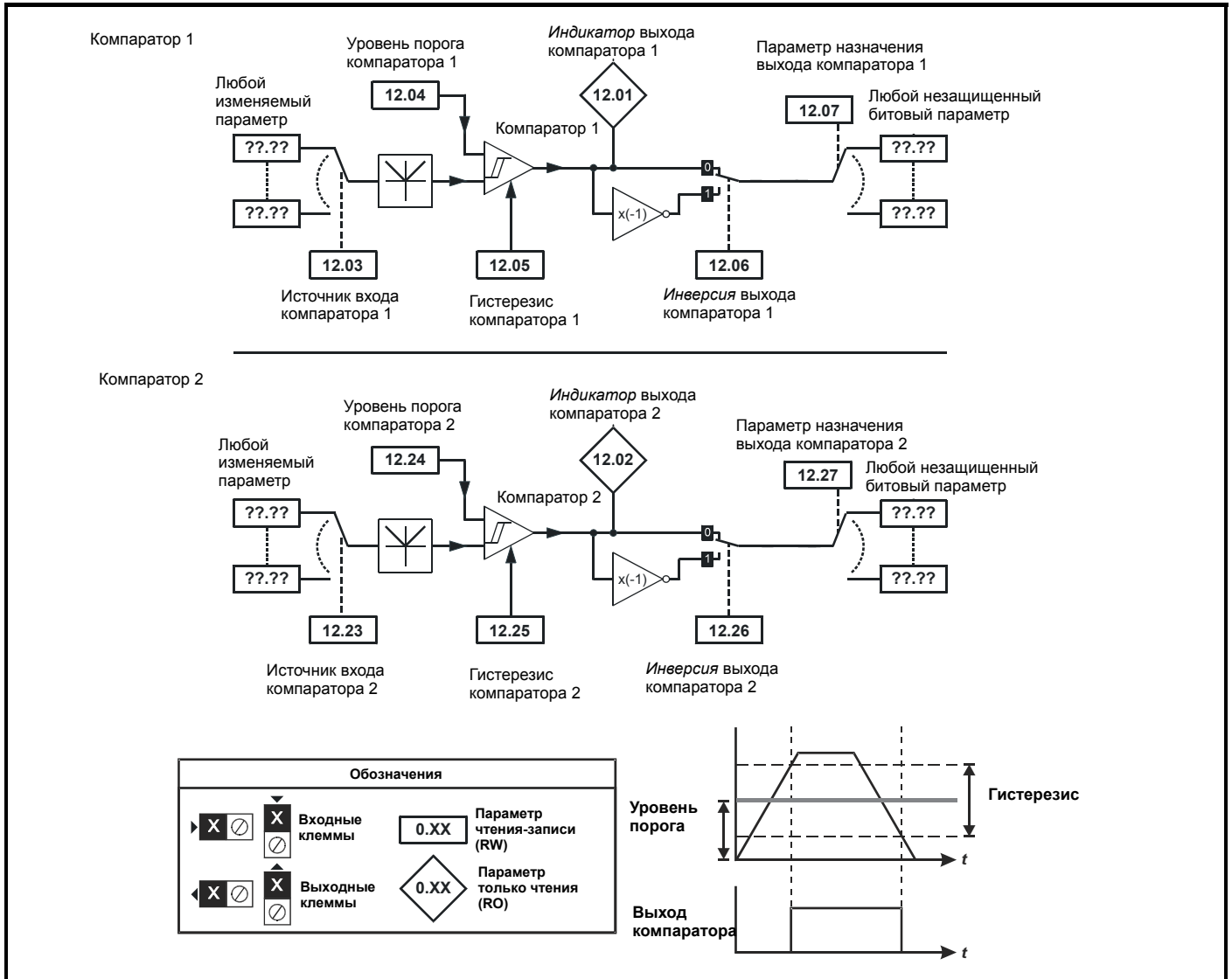
Рис. 11-14 Логическая схема Меню 12
