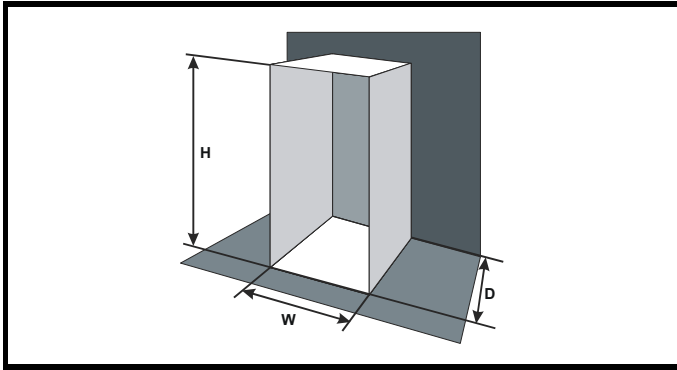
Рис. 3-22 Шкаф, в котором верхняя, передняя и боковые панели могут рассеивать тепло
