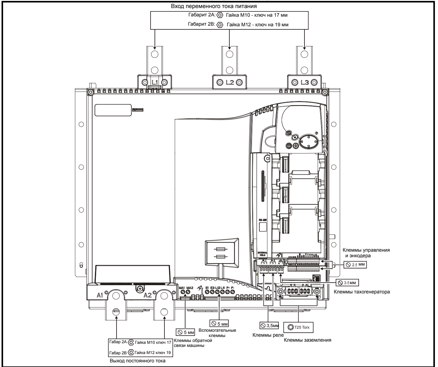
Рис. 3-24 Расположение клемм питания и заземления на электроприводах габарита 2А и 2В
