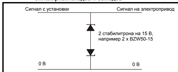
Рис. 4-15 Подавление выбросов для аналоговых и биполярных входов и выходов
