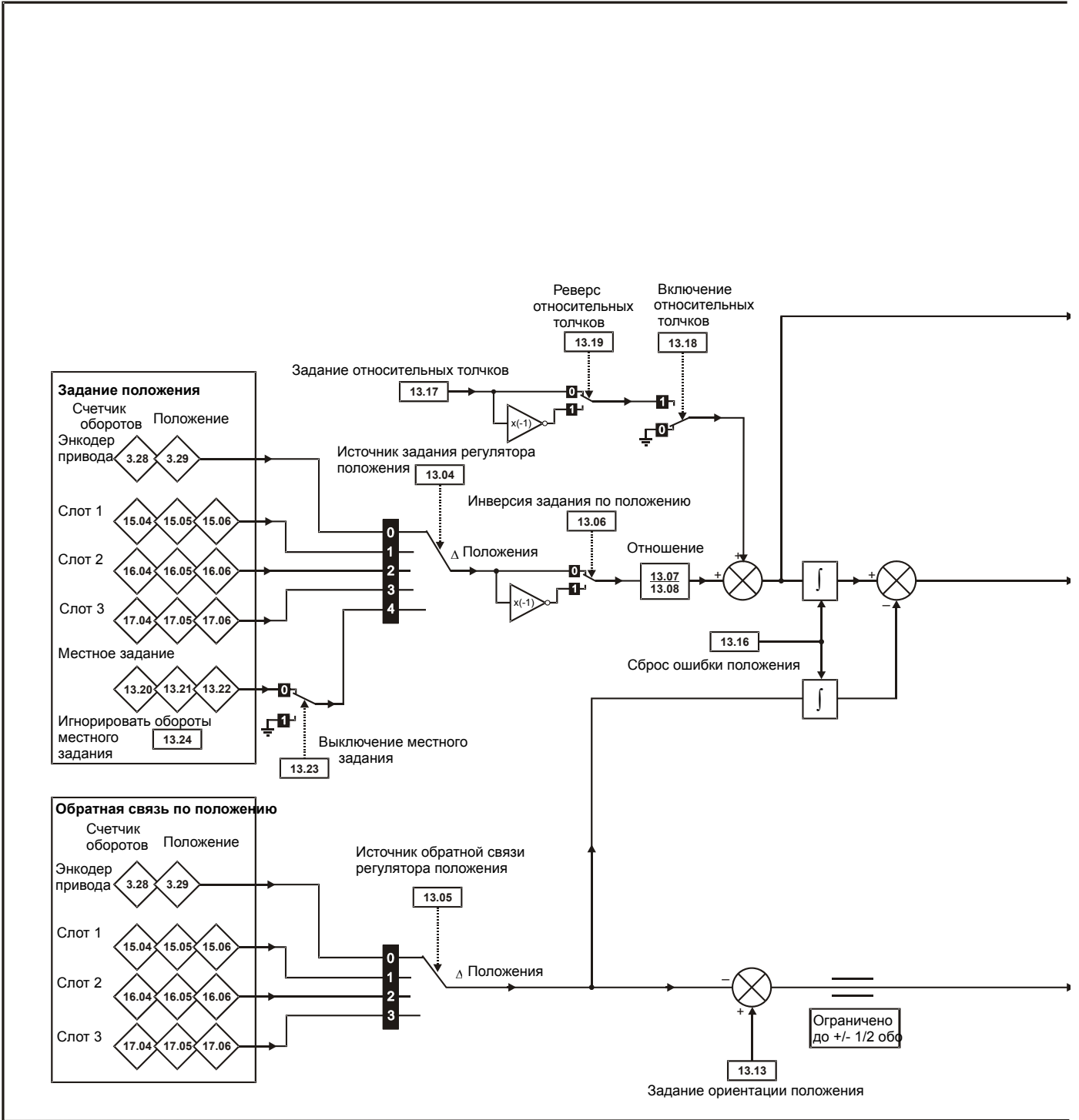
Рис. 11-18 Логическая схема Меню 13
