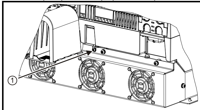
Рис. 4-7 Отсоединение перемычки между заземлением и варистором на электроприводах габарита 2А / 2В
