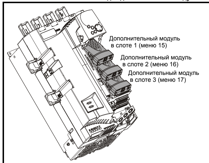
Рис. 11-20 Расположение слотов для дополнительных модулей и соответствующие им номера меню
