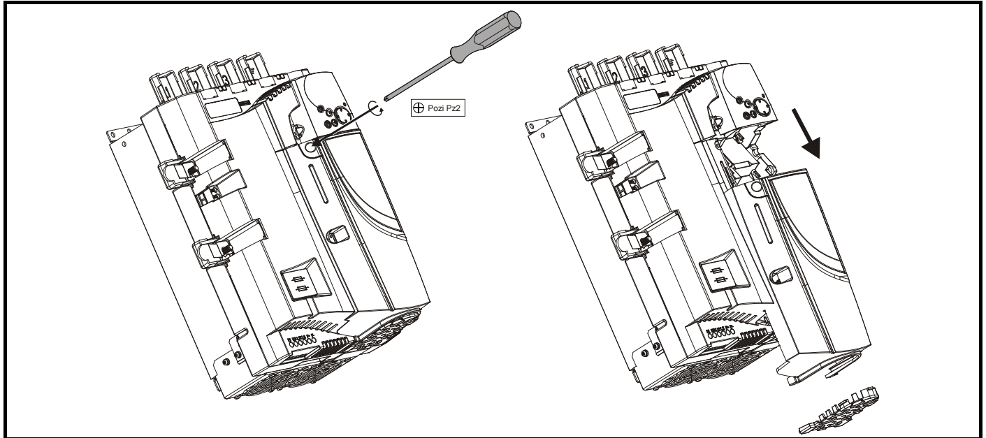
Рис. 3-3 Снятие крышки клемм управления (показан габарит 1)
