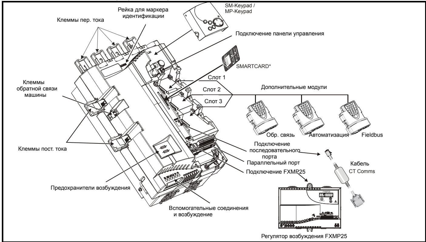
Рис. 2-5 Общий вид и опции электропривода габарита 2
