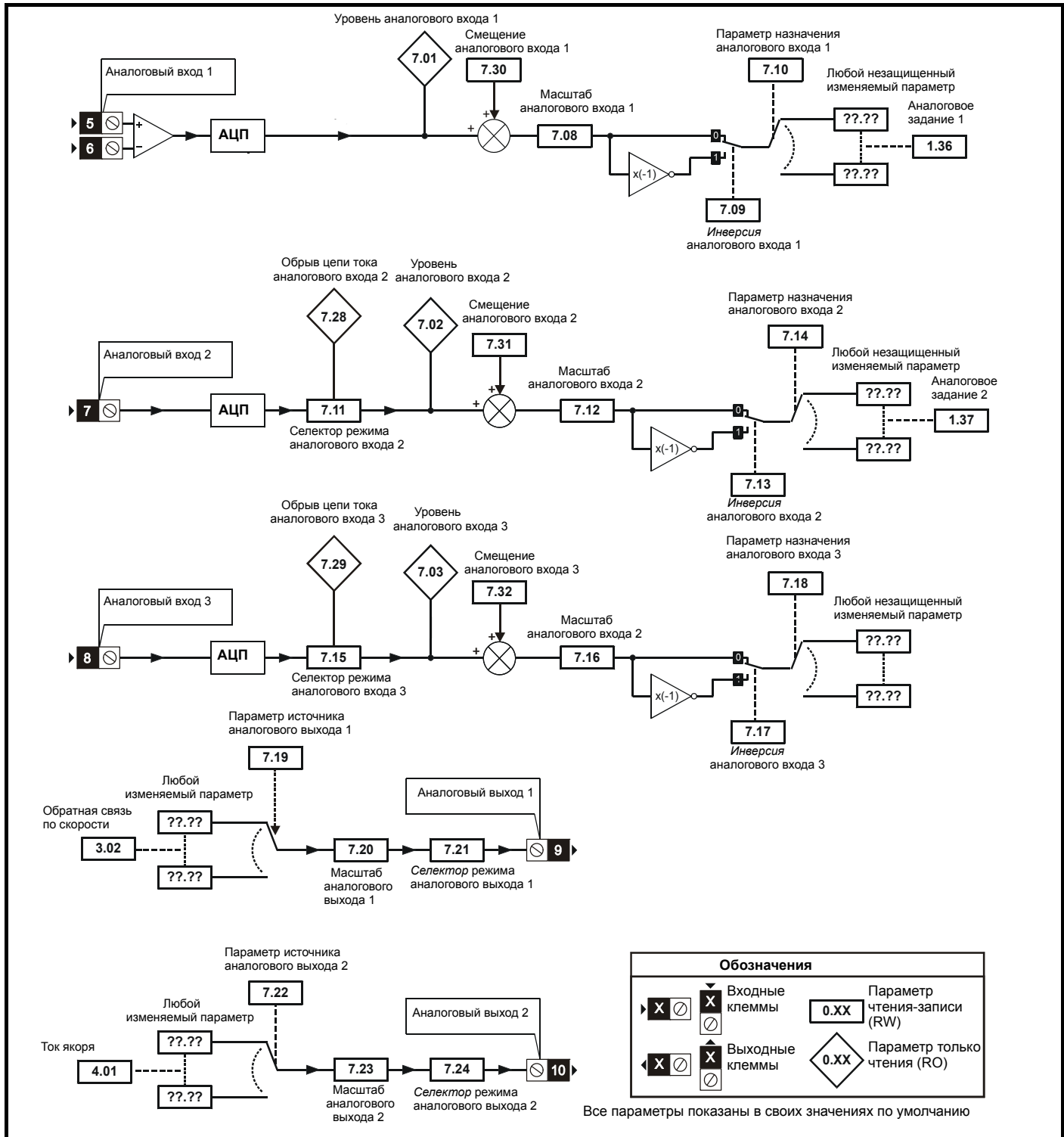
Рис. 11-8 Логическая схема Меню 7
