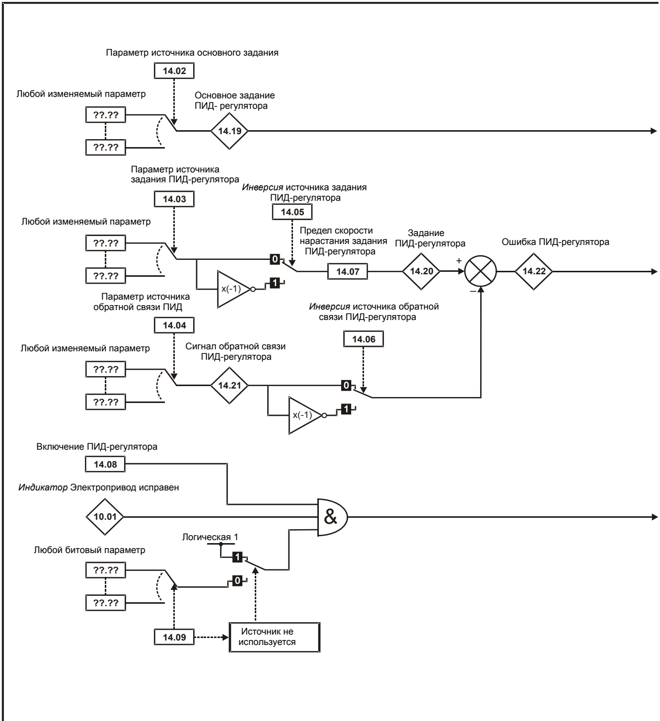
Рис. 11-19 Логическая схема Меню 14
