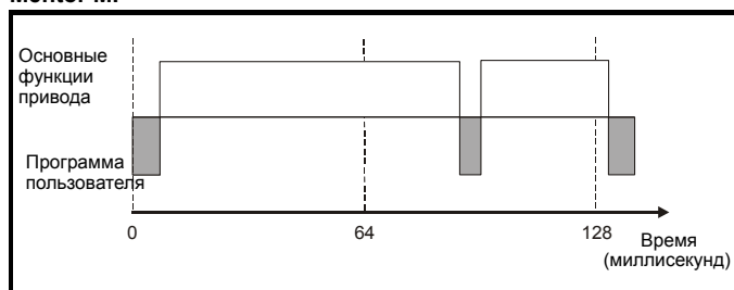
Рис. 10-1 Диспетчеризация программы встроенного ПЛК в Mentor MP
