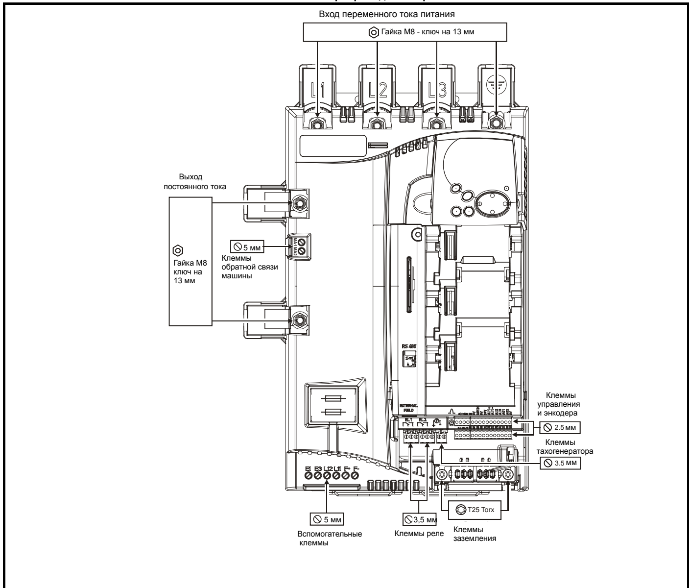
Рис. 3-23 Расположение клемм питания и заземления на электроприводах габарита 1
