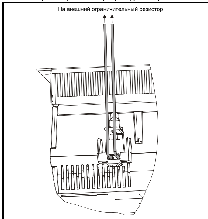
Рис. 4-11 Размещение клемм внешнего ограничительного резистора на электроприводах габарита 2
