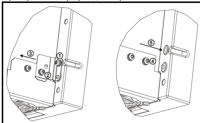
Рис. 4-6 Отсоединение перемычки между заземлением и варистором на электроприводах габарита 1
