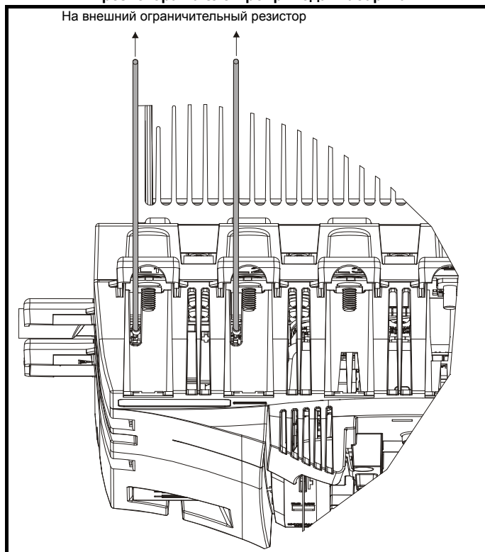
Рис. 4-11 Размещение клемм внешнего ограничительного резистора на электроприводах габарита 2
