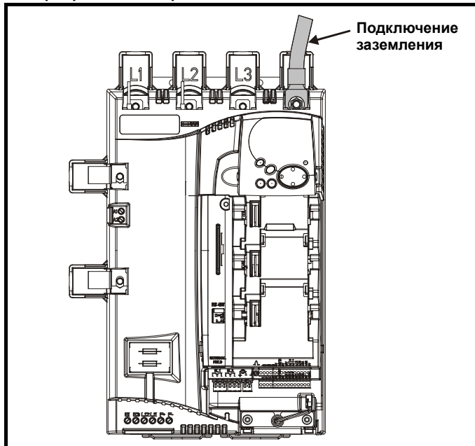
Рис. 4-4 Расположение подключения заземления на
