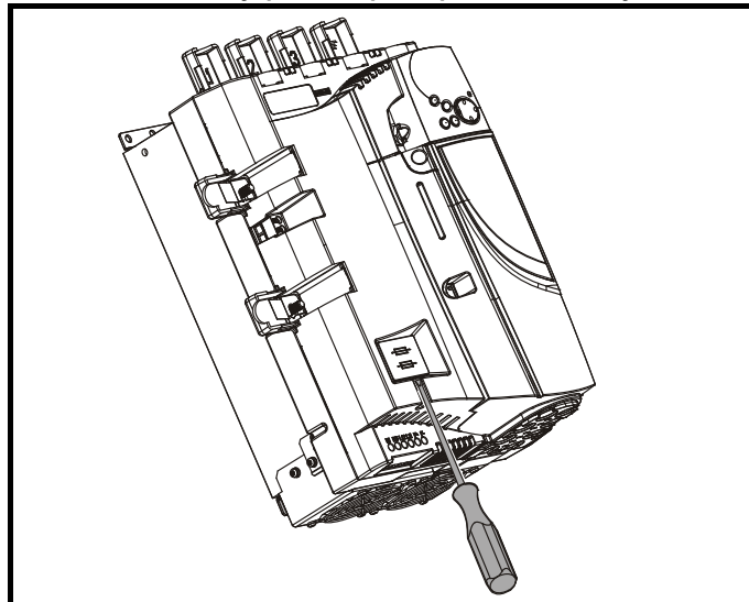
Рис. 4-9 Снятие внутренних предохранителей возбуждения
