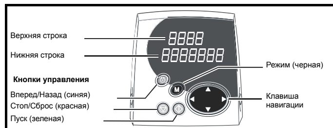
Рис. 5-1 SM-Keypad
