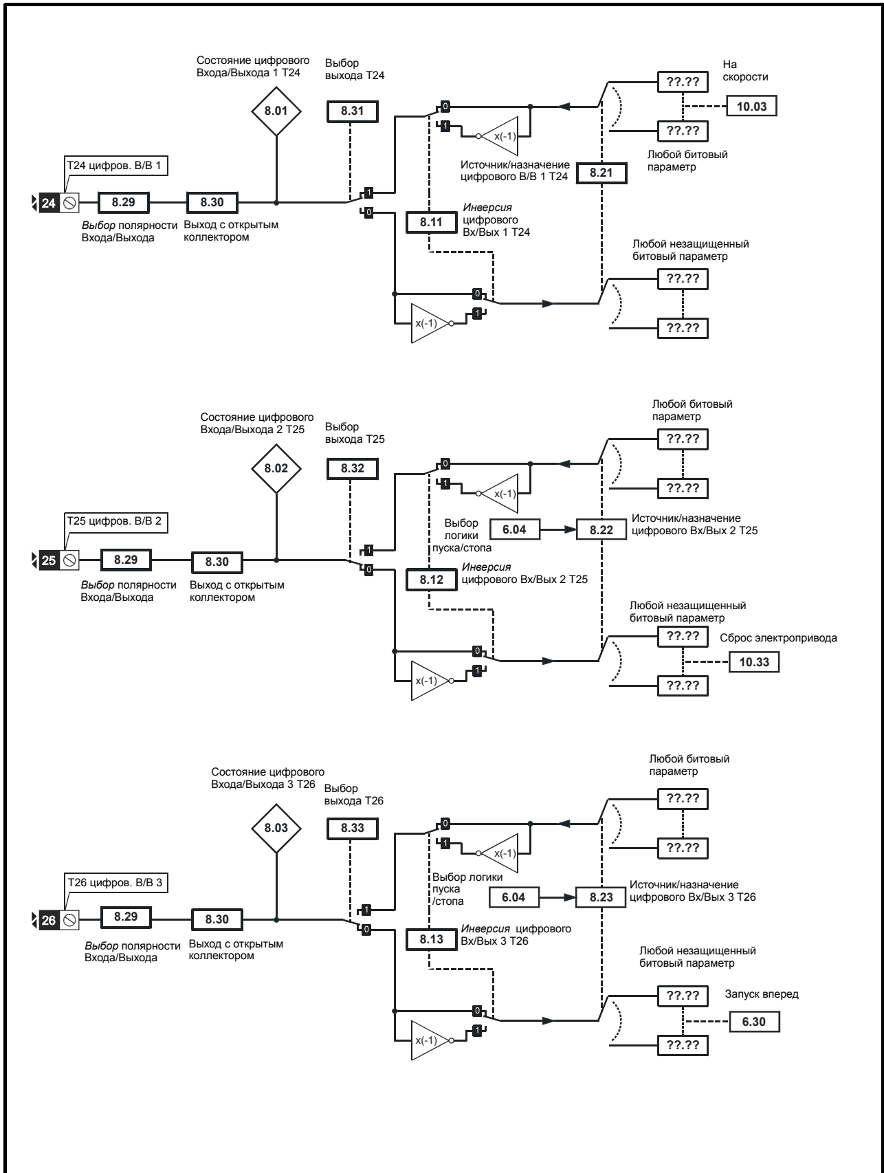
Рис. 11-9 Логическая схема Меню 8
