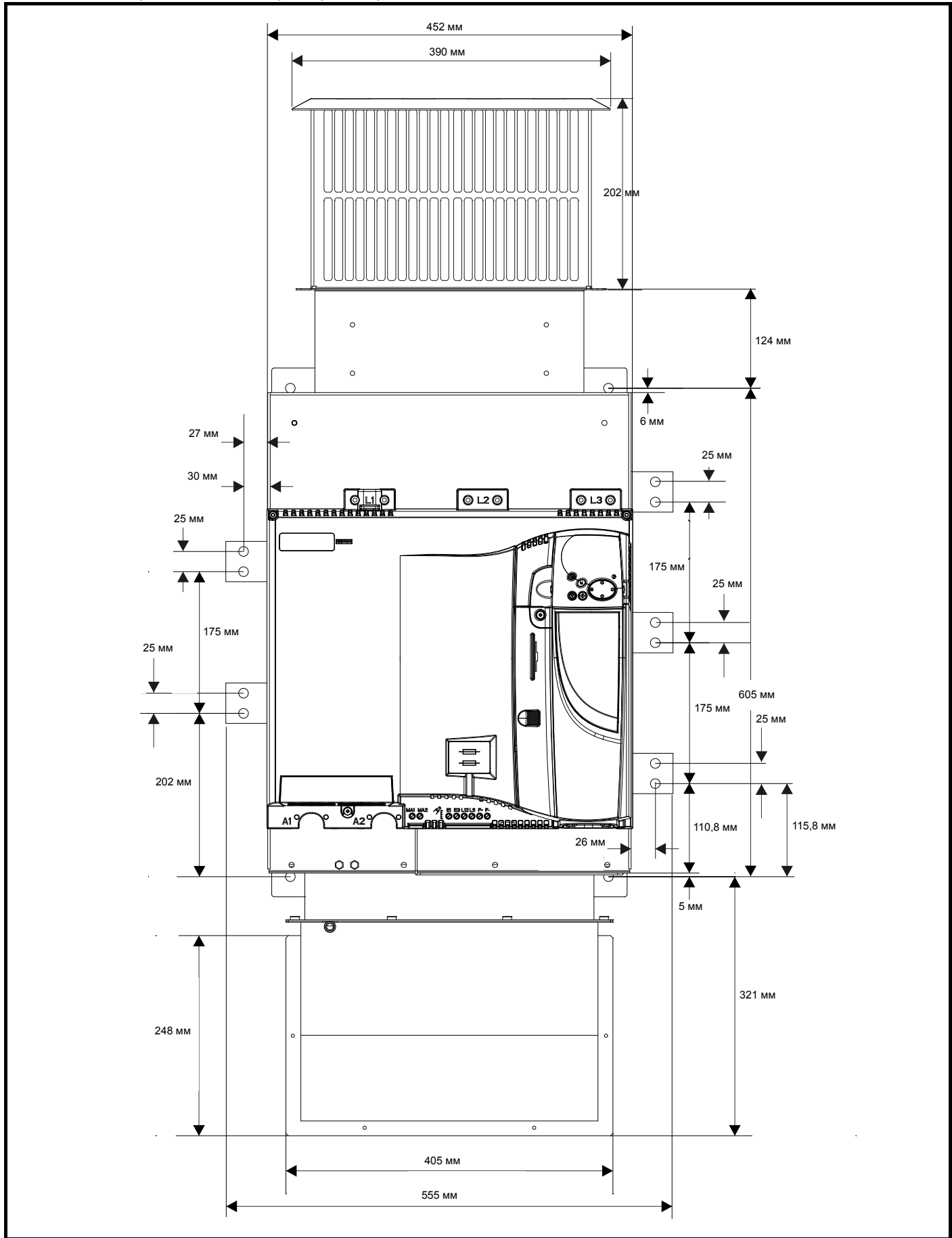
Рис. 3-13 Вид спереди и монтажные размеры габарита 2С
