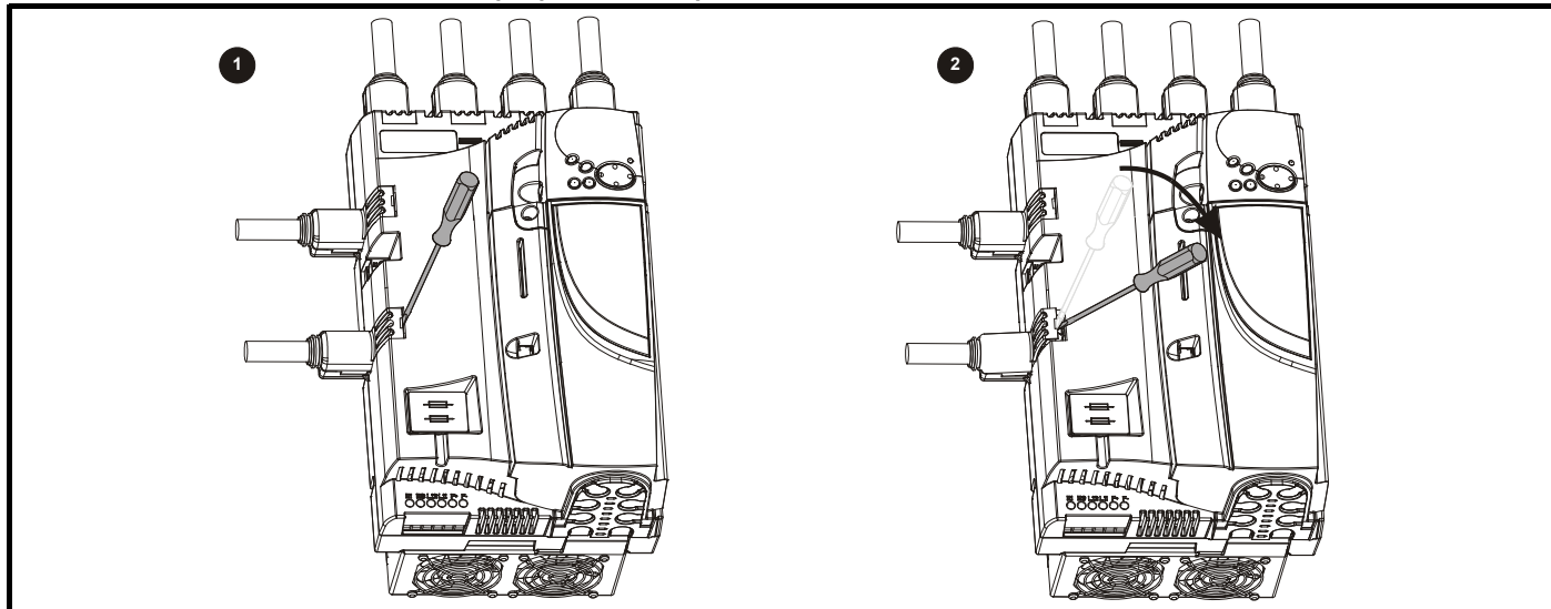
Рис. 3-19 Снятие чехлов клемм на электроприводах габарита 1
