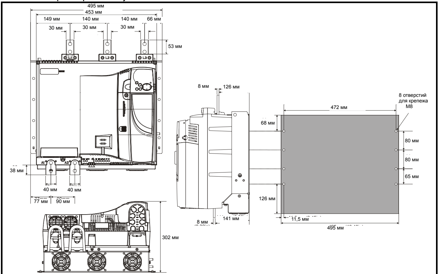
Рис. 3-12 Размеры габарита 2B без установленных чехлов клемм
