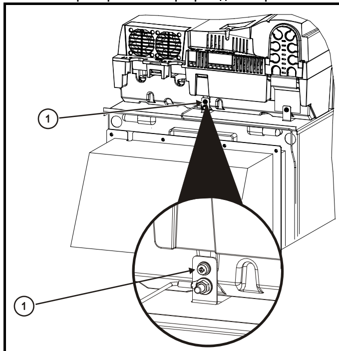
Рис. 4-8 Отсоединение перемычки между заземлением и варистором на электроприводах габарита 2С / 2Д
