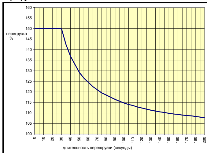
Рис. 12-1 Максимальная допустимая длительность перегрузки
