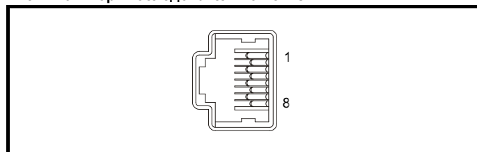
Рис. 4-16 Порт последовательной связи
