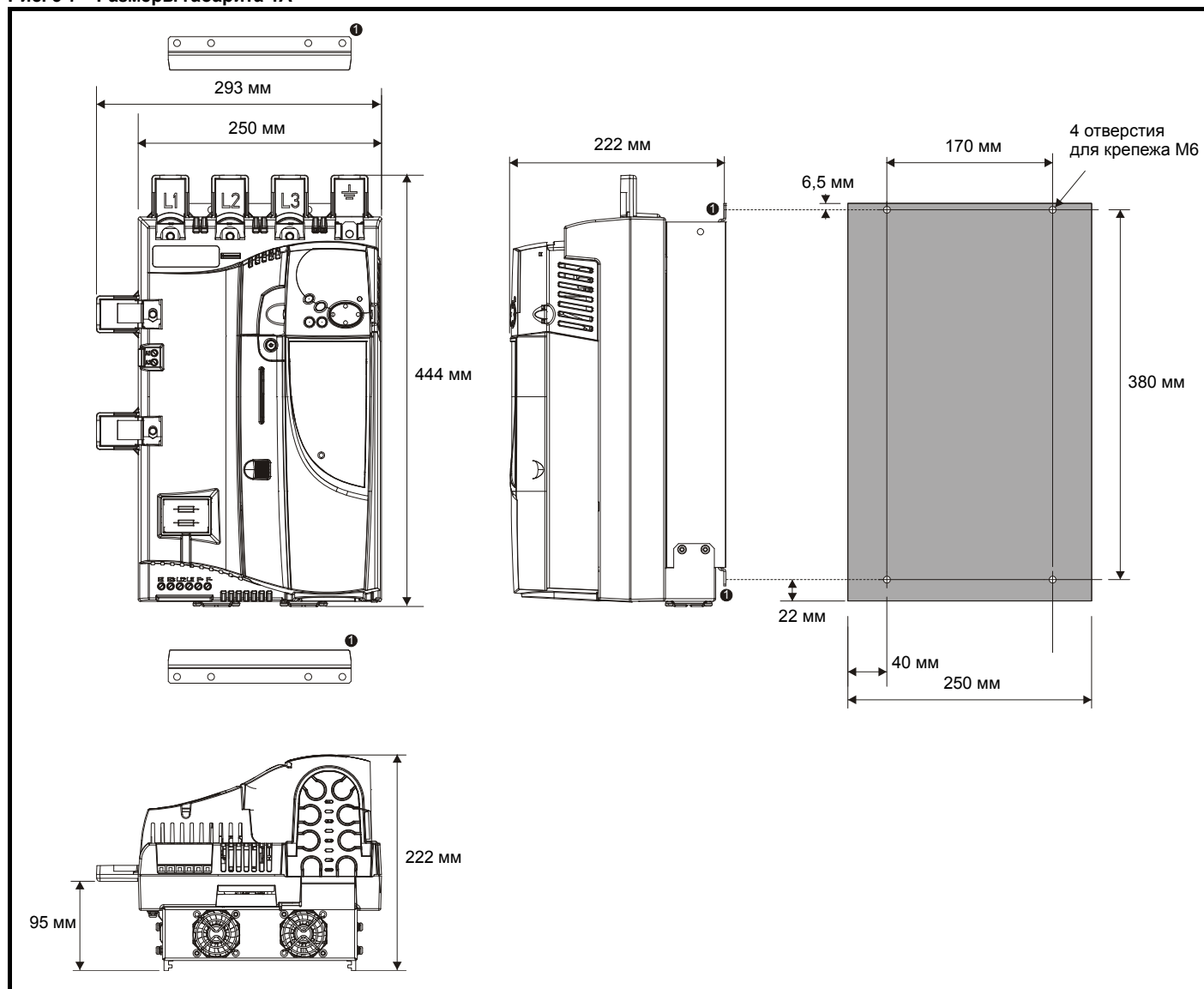
Рис. 3-7 Размеры габарита 1А
