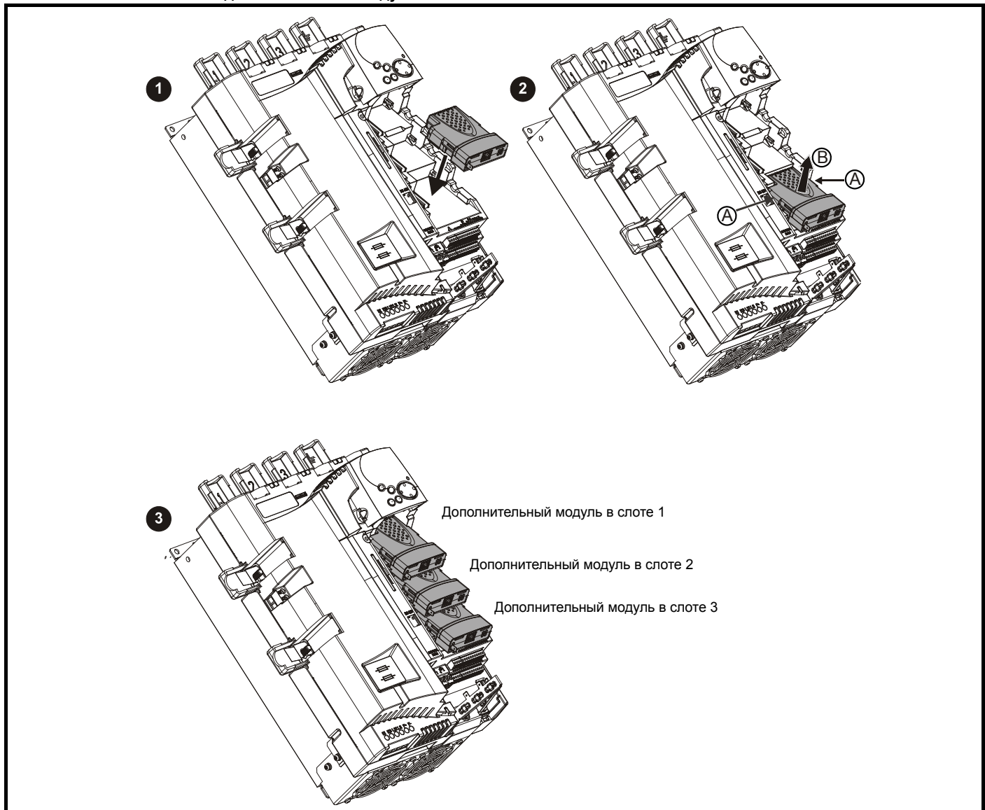
Рис. 3-5 Установка и снятие дополнительного модуля
