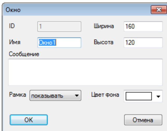
Рисунок 3.11 – Свойства окна
