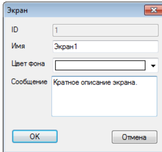
Рисунок 3.10 – Свойства экрана
