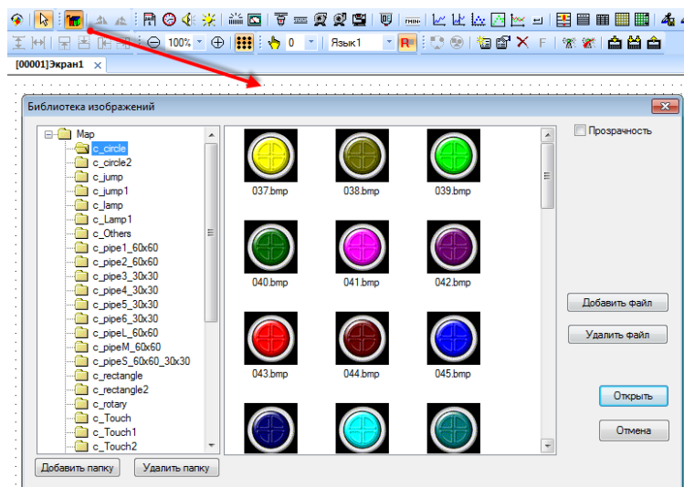
Рисунок 3.37 – Библиотека элементов
